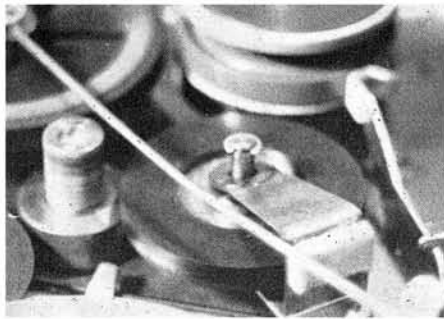
Fig. 2 Idler return spring
