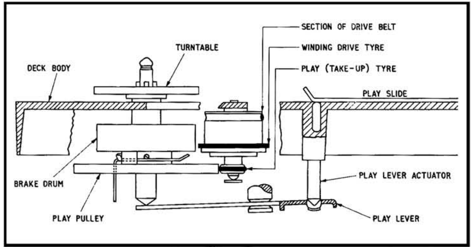
Fig. 8. Ampex 753 arrangement.
