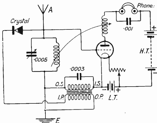
FIG. 2. TRINADYNE CIRCUIT
