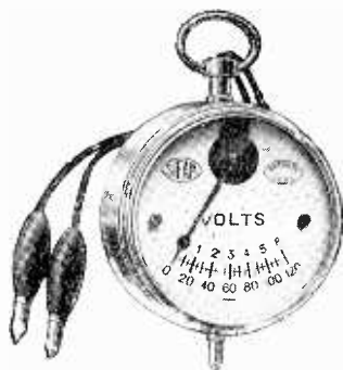
FIG. 25. THE SIFAM COMBINED H.T. AND L.T. VOLTMETER
