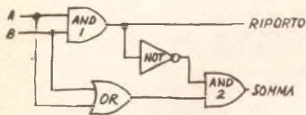
Fig. 4 - Impianto logico del circuito XOR.
