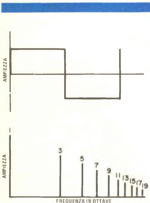
Fig. 2 - Parte dello spettro di un'onda quadra perfetta.
