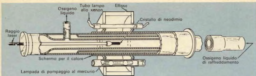
Nei laser a cristallo ad onda continua si usa una disposizione delle parti simile a quella adottata per la realizzazione di questo progetto della Bell. Il cristallo di neodimio è situato in un fuoco della cavità ellittica, mentre nell'altro fuoco si trova la lampada al mercurio che pompa la luce.
