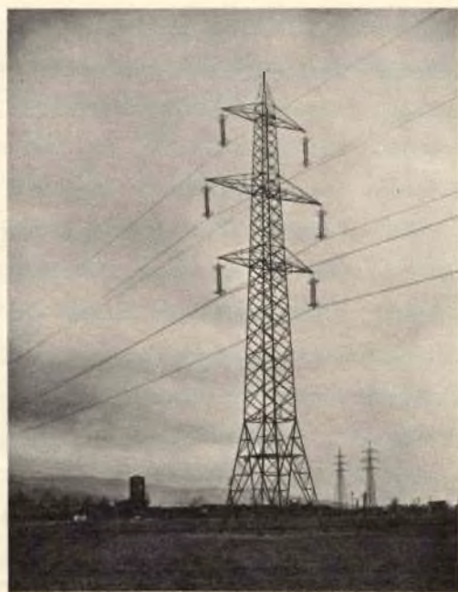
La linea Turbigio 2° da 220 kV della SIP unisce la Lombardia al Piemonte. E' chiaramente visibile la fune di guardia installata in cima al traliccio per proteggere la linea da possibili fulminazioni.
