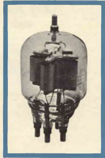
Questo è un tipico tubo trasmittente costruito dalla Westinghouse. La placca del tubo è di grafite.
