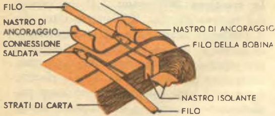
Fig. 5 - Sistema per effettuare le prese sui secondari in modo da realizzare uguali reattanze di dispersione.
