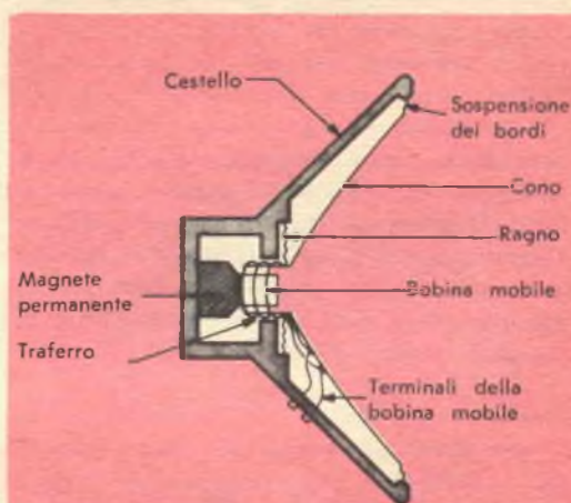
Fig. 1 - Sezione di un tipico altoparlante a magnete permanente. Il circuito magnetico rappresenta il « motore » e il cono è il « pistone » che fa muovere l'aria.
