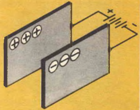
Fig. 3 - In A è rappresentato il principio fondamentale di funzionamento dell'altoparlante elettrostatico. Quando le armature hanno cariche di uguale segno si respingono, e quando le cariche sono di segno opposto si attraggono. In B si vedono i collegamenti di un altoparlante elettrostatico.
