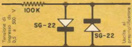
Fig. 4 - Circuito limitatore di volume a stabistori.
