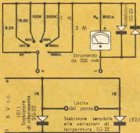
Fig. 3 - Ponte a stabistori sensibile alla temperatura, che dà, al variare di questa, una variazione lineare del potenziale in uscita. La tensione di alimentazione del ponte può variare del 20% pur mantenendo costante la tensione in uscita.
