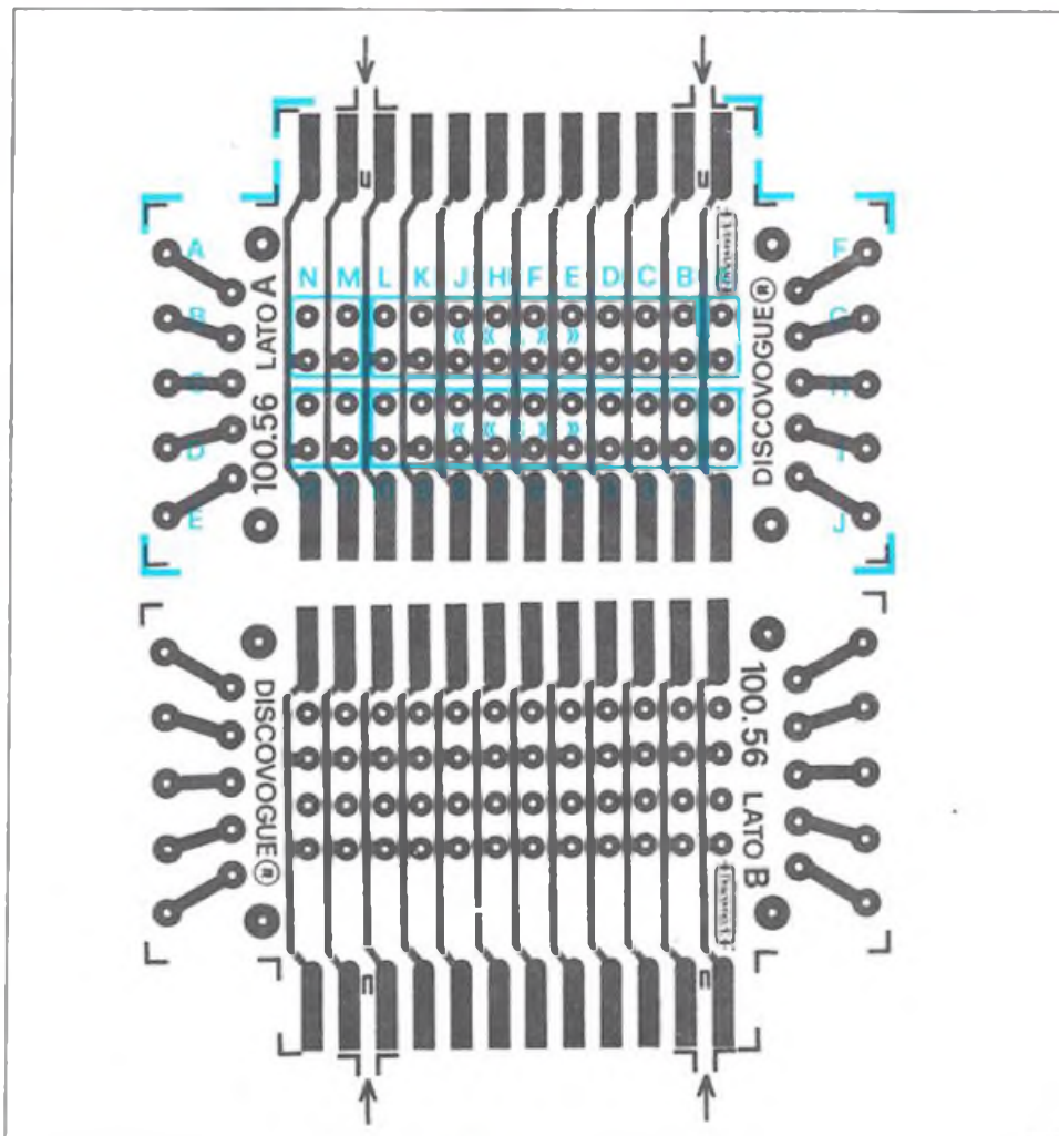
Figura 3. Piste conduttrici del lato A e B del circuito stampato cod. 100.56 con montaggio dei componenti sul lato A.
