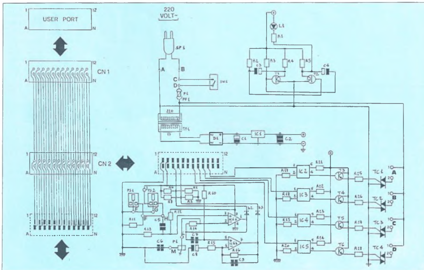
Figura 1. Schema circuitale.
