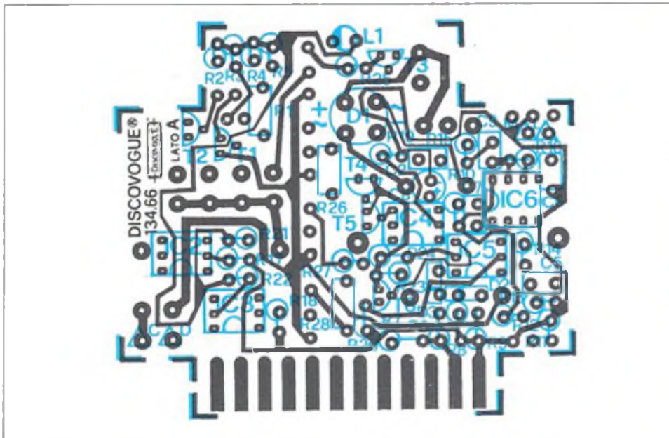
Figura 4. Pista conduttrice del lato A del circuito 134.66 con montaggio dei componenti sul lato A.
