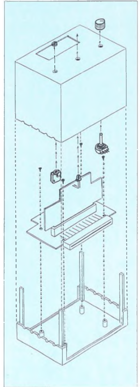
Figura 6. Inserimento del circuito nel contenitore.
