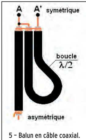
5 - Balun en câble coaxial.
