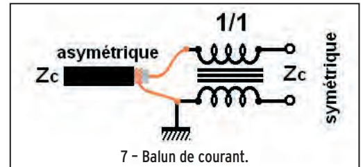
7 - Balun de courant.
