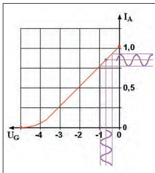
Figure 6 : Courant d'anode en fonction de tension grille.
