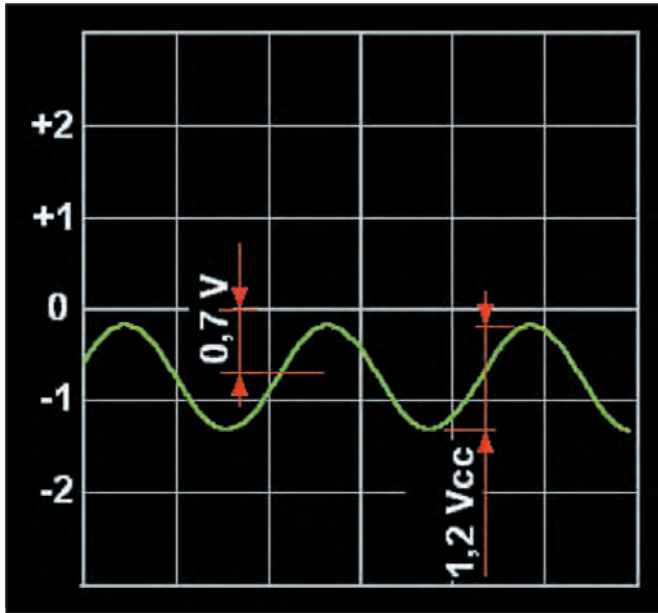
Figure 3 : Ce que l'on peut voir sur la grille d'une triode.
