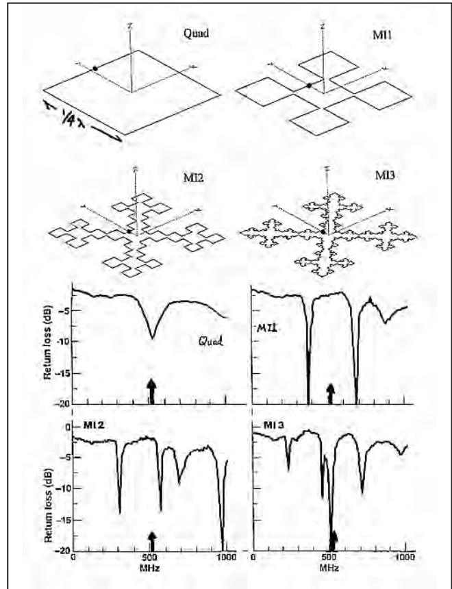
Figure 9 : Fractalisation d'une boucle réalisée par Nathan Cohen NIIR.
