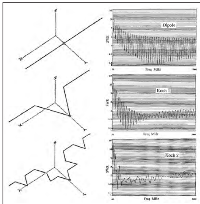
Figure 10 : Fractalisation d'un dipôle réalisée par Nathan Cohen NIIR.
