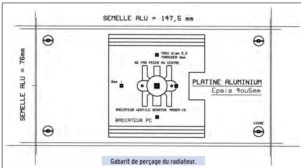
Implantation de l'ampli 30W.
