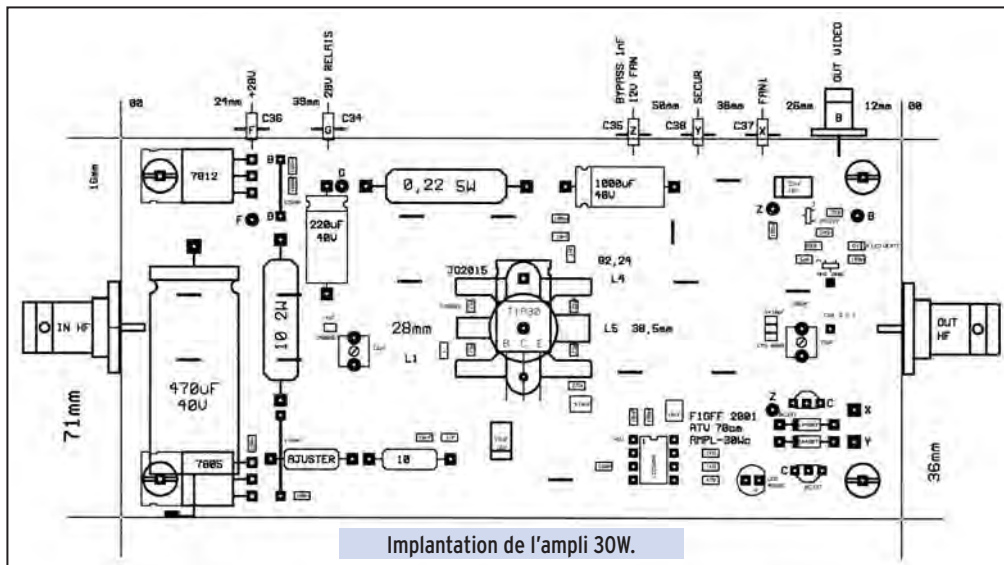
CI de l'ampli 30W.
