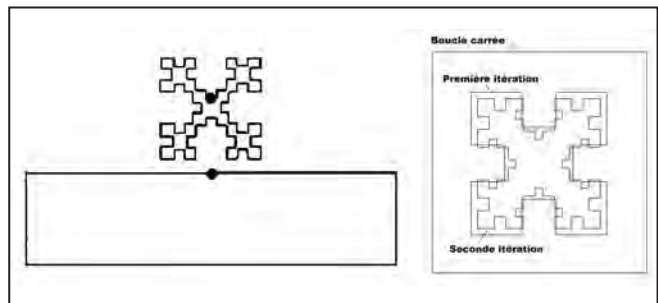
Figure 6 : A gauche : Dimensions comparées de deux boucles de mêmes caractéristiques, avant et après fractalisation. A droite : En ajoutant des itérations, on réduit les dimensions de l'élément, pour une fréquence donnée.
