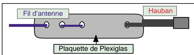
▲ Figure 3 : Isolateur vu de profil.
