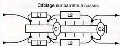
Câblage sur barrette à cosses
