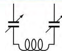
Fig. 3b : Accord en série.
