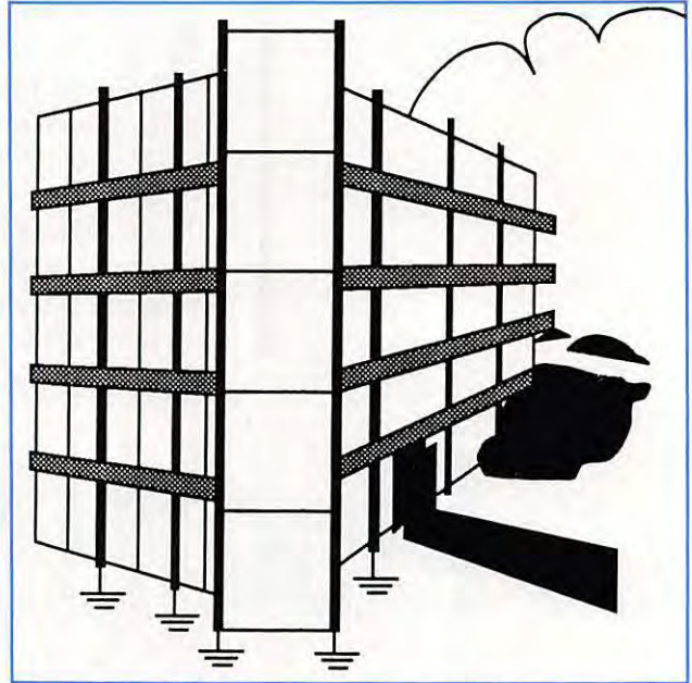
Paratonnerre à cage maillée.
