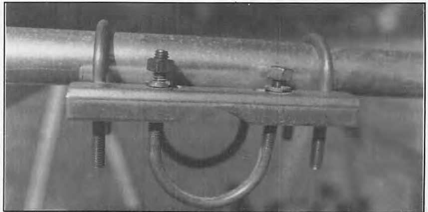
Fixation des brins rayonnants sur le boom.
