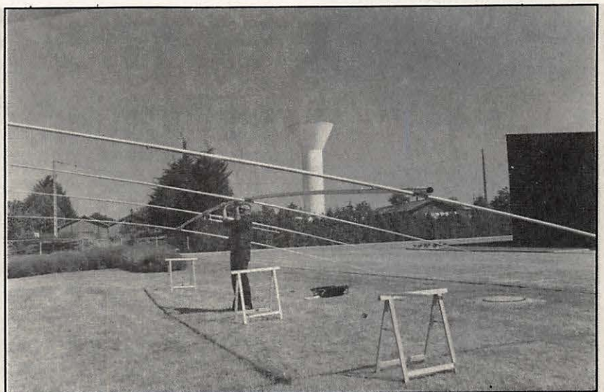
Des tréteaux pour le montage et le réglage. Ici, F3TA, portant l'antenne.
