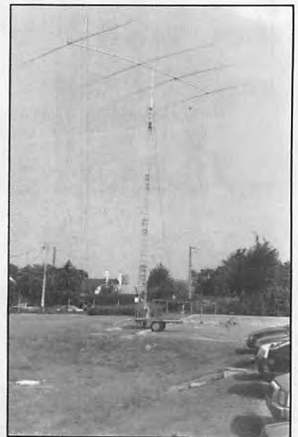
L'antenne est montée.
