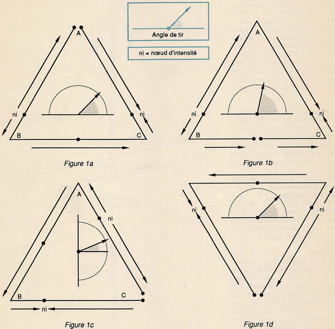
Figure 1 : Propriétés de la Delta-Loop verticale
