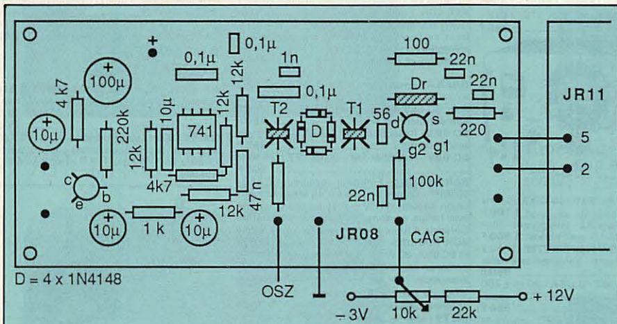
Figure 2 : Implantation des composants (échelle approximative)
