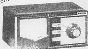
Prix : 1183 ▲ DAIWA - CN 620. Wattmètre à aiguilles croi- sées, 1,8 à 150 MHz, 20 W/200 W/2 kW.
