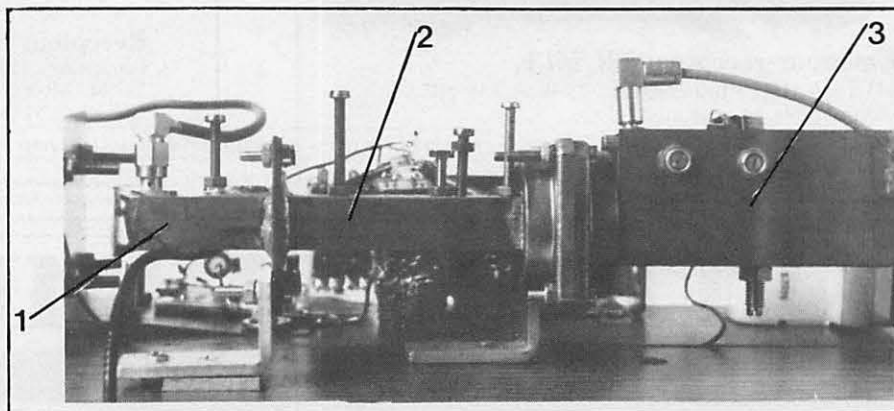
Photo 4 : Multiplicateur Mélangeur 10 224 / 10 368 MHz
