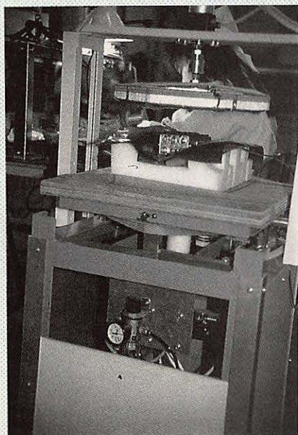
Banc testant la résistance aux vibrations.
