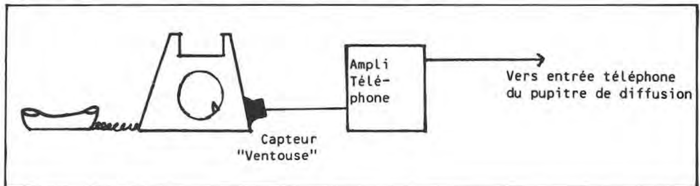
Synoptique n° 7
