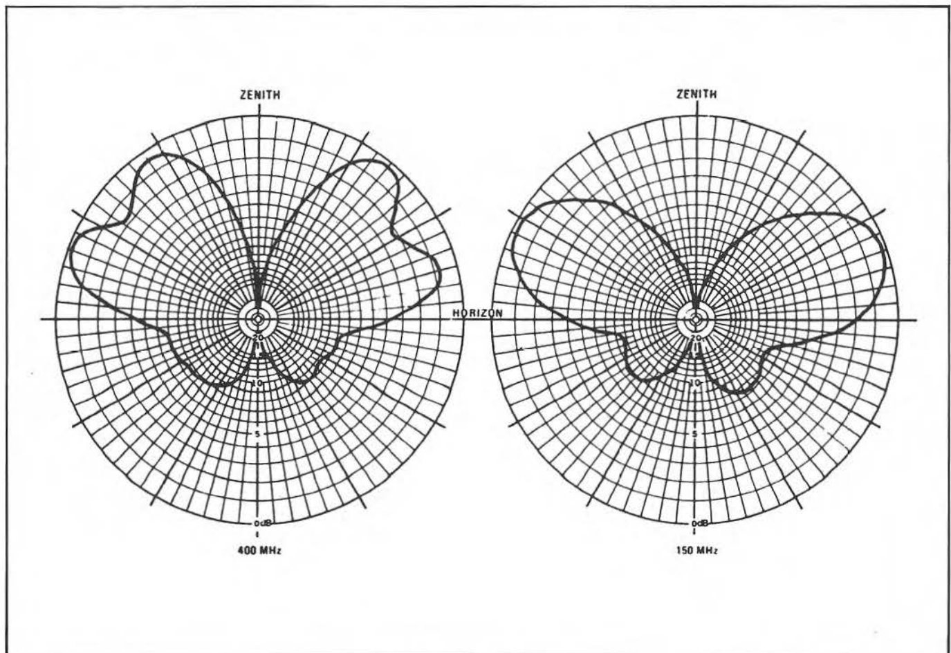
Figure A — Diagramme de réponse d'antenne Récepteur MAGNAVOX MX 1502
