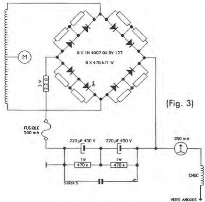
ALIMENTATION HAUTE-TENSION
