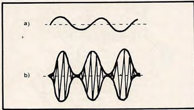
Figure 9 Représentation sur un tube d'oscilloscope d'un signal HF modulé à 100 %.
