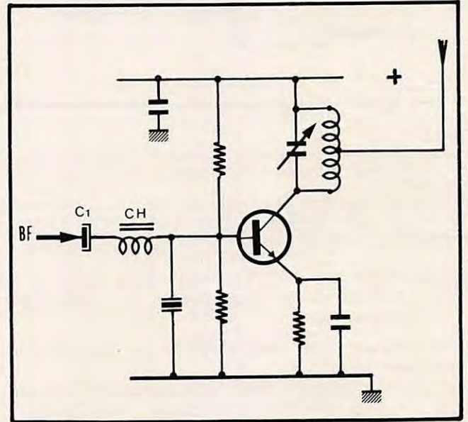
Figure 11 Du fait que le courant collecteur dépend du courant base, il existe la possibilité d'effectuer une certaine modulation d'amplitude en appliquant le signal BF directement sur la base du transistor oscillateur.
