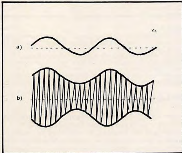
Figure 10 Représentation graphique d'une modulation à 40 % environ.
