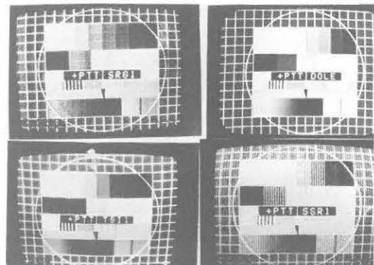
En haut, à gauche, mire électronique couleur PAL type FUBK captée à Rennes le 22 juillet 80 de 13h30 à 14h15 UTC. Canal E2. En haut, à droite, mire de diffusion PTT La Dôle, émise par un générateur de mire électronique couleur PAL. Prise à Genève La Dôle. En bas, à gauche, même type de mire, canal 34 UHF, puissance 100kw PAR. Photo prise près du centre émetteur de la Dôle lors de la visite. En bas, à droite, même type de mire captée à Rennes le 10/9/78 canal E4 VHF bande 1 de 7h05 à 7h30 UTC.
