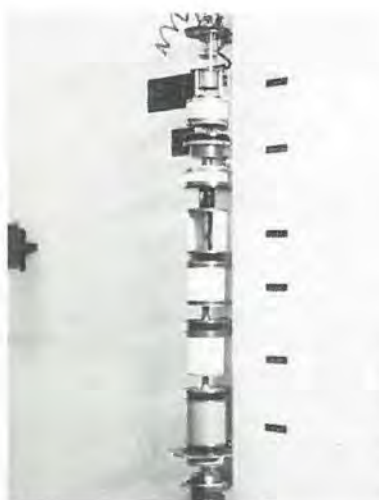
Vue du coeur d'un Klystron comprenant : la cathode l'anode la 1ère cavité la 2ème cavité la 3ème cavité etc.....
