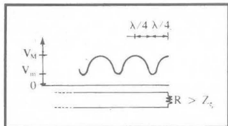
Fig. B.3.3c. Ondes stationnaires fournies par le battement d'une onde directe V_d et d'une onde réfléchi V_r dans le cas où R > Z_c : on a un ventre de tension sur la charge (nœud de courant).
