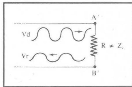
Fig. B.3.3b. L'énergie refusée par la charge provoque une onde progressive réfléchi V_r plus petite que V_d .
