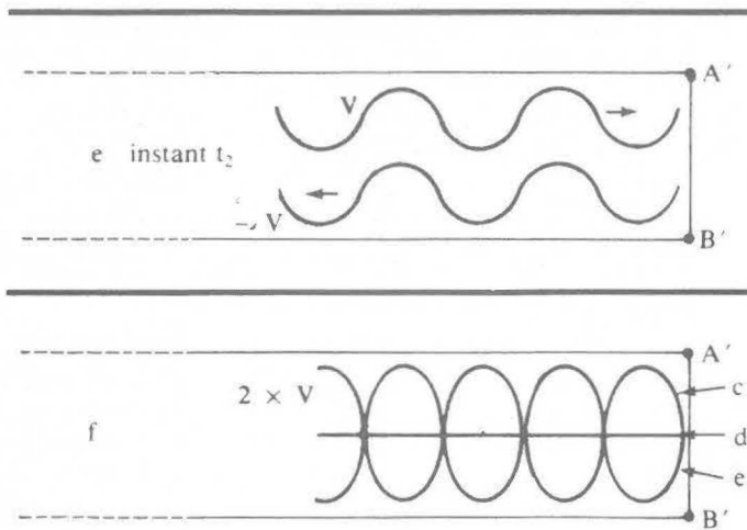
Fig. B.3.2c, d, e et f. Allure des ondes directe et réfléchi à trois instants successifs t_0 , t_1 et t_2 (ligne en court-circuit). En bas, la tension obtenue en ajoutant algébriquement point par point ces tensions directe et réfléchi.
