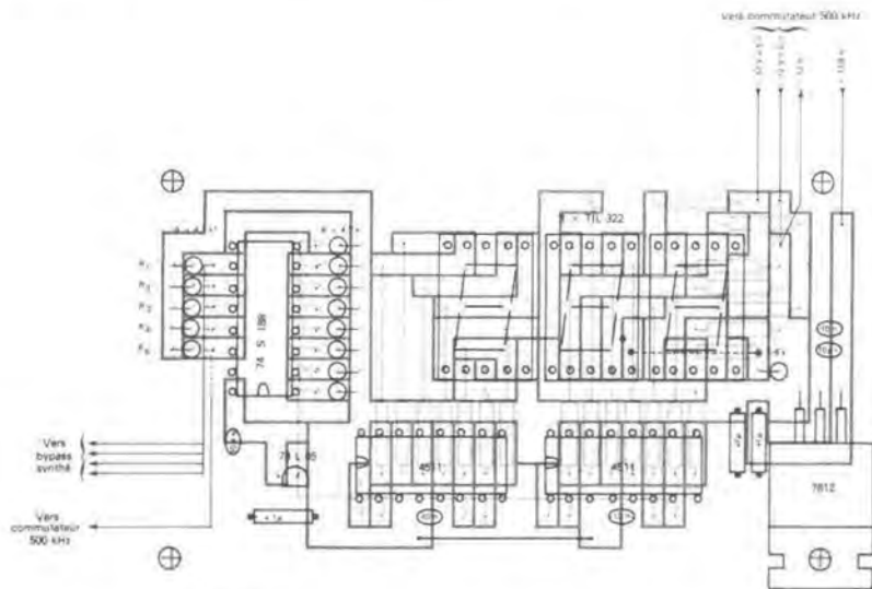
* Voir texte Fig. 6. IMPLANTATION DES COMPOSANTS (CÔTÉ ÉPOXI).
