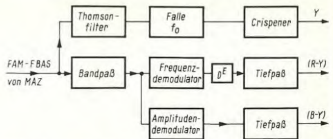
Bild 2. Demodulation des FAM-Signals. Die verwendeten Systemparameter sind in der Tabelle angegeben
