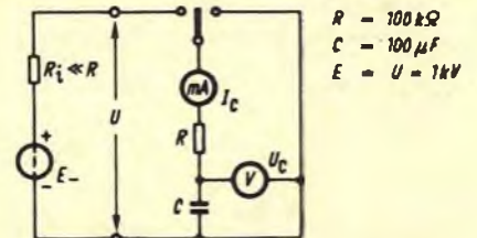
Bild 3.5. Messschaltung zur Aufnahme der Lade- und Entladekurven eines Kondensators
