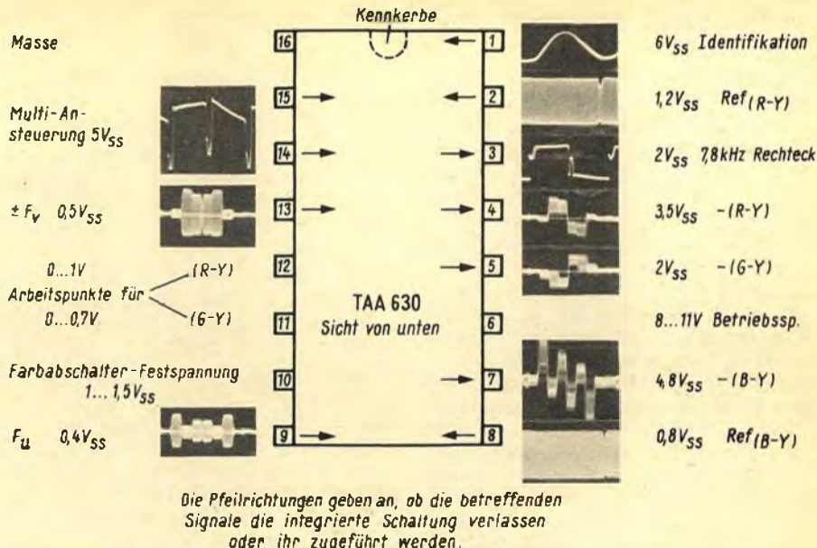
Bild 4. Anschlußschema der IS mit Spannungangaben und Oszillogrammen
