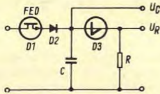
Bild 7. Treppenspannungsgenerator als Impulsteiler am Ausgang U_R
