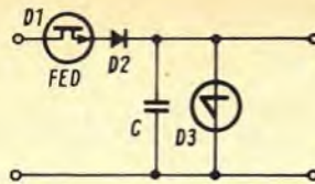
Rechts: Bild 6. Treppenspannungsgenerator mit FE-Diode
