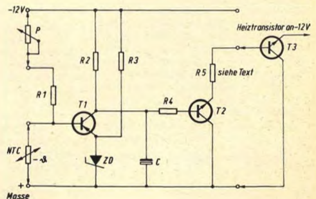
Bild 1. Schaltung des kontaktlosen Thermostaten
