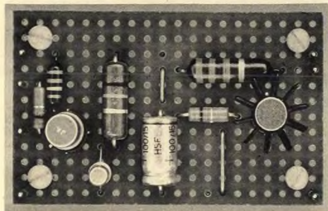
Unten: Bild 2. Aufbau des kontaktlosen Thermostaten. Links: Platine des Mustergerätes; rechts: Bestückungsplan (siehe auch Strickliste)
