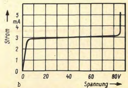
Bild 2. Kennlinien einer Feldeffektdiode (nach Motorola); a = grundsätzlicher Verlauf, b = Kennlinie des Typs MCL 1303 mit I_D = 3,0 mA
