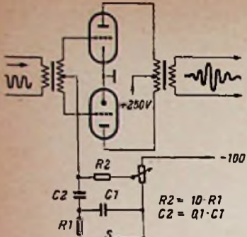
Bild 2. Schaltung des Impulsgebers
