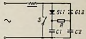
Schaltung zur Funkenlöschung für den Schalter S
