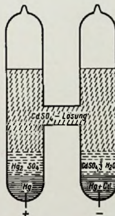
Bild 1. Das Internationale Weston-Element als Spannungsnormal
