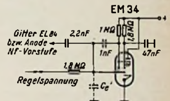
Bild 3. Schaltung zur Rauschunterdrückung im UKW-Bereich mit EM 34
