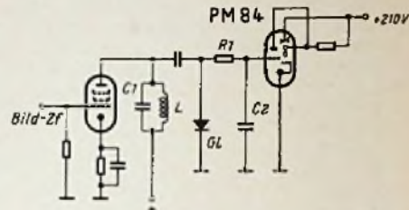
Bild 11. Prinzipschaltung der Abstimmmanzeige mit dem Magischen Band
