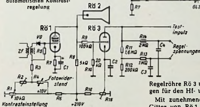
Unten: Bild 2. Prinzip der automatischen Kontrasteinstellung
