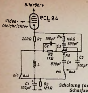
Bild 3. Schaltung für Weich- und Scharfzeichnung
