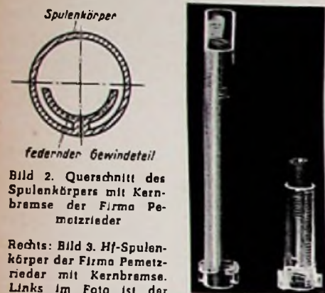
Bild 2. Querschnitt des Spulenkörpers mit Kernbremse der Firma Pemetzrieder
