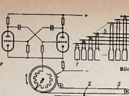
Bild 3. Prinzip des Glissando-Multivibrators
