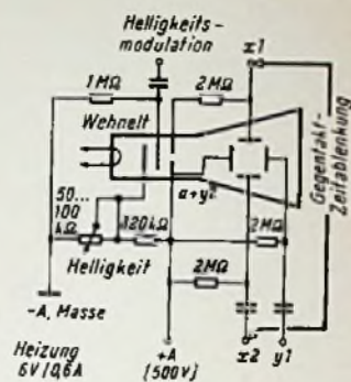
Bild 2. Prinzipschaltung einer Röhre 1 CP 1
