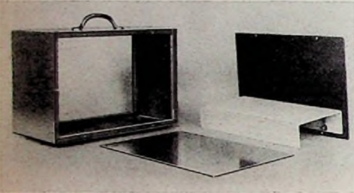
Oben: Bild 1. Bestandteile für ein selbstgebautes Gehäuse. Sehr zweckmäßig erweisen sich Vierkant-Aluminiumstangen für die Rahmen innerhalb der Zarge und U-Profil für das Chassis
