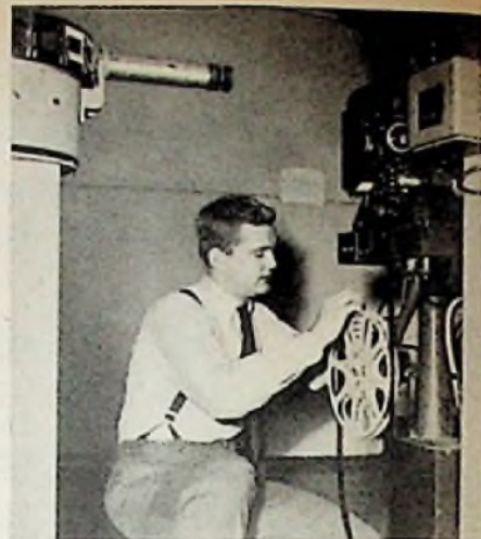
Bild 2. Einlegen eines 16-mm-Filmes in den Filmprojektor im Filmraum von AFR-TV. Der links sichtbare Dia-Abtaster wird ebenso wie der Filzaabtaster vom Kontrollraum aus ferngesteuert
