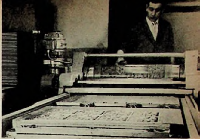
Bild 1. Mit dieser Offset-Presse werden die Schaltungen auf die kupferkascherten Platten mit einer ätzfesten und lötfähigen Farbe gedruckt
