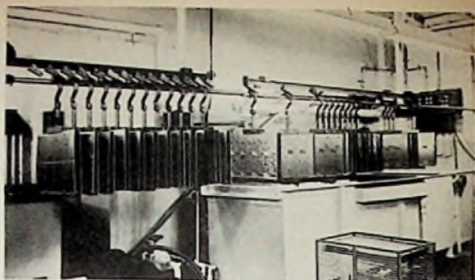
Bild 6. Vollautomatische Ätzanlage. Die mit ätzfester und lötfähiger Farbe bedruckten Platten werden geätzt, gespült und gemässort. Der letzte Arbeitsvorgang in dieser Etappe ist die Trocknung
