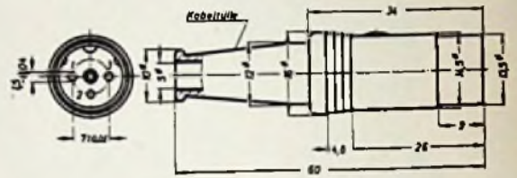
Nr. 5991 Zwerg-Stecker 3 polig
