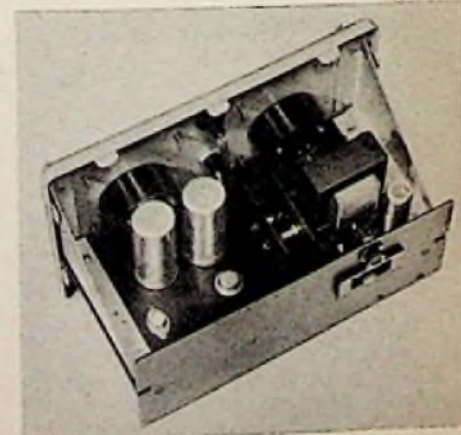
Bild 7. Labormuster des von Valvo entwickelten transistorgeregelten Netzgerätes; oben = Vorderansicht ohne Gehäuse, unten = Aufsicht auf das Chassis
