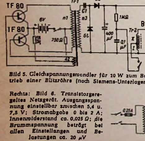
Bild 5. Gleichspannungswandler für 10 W zum Betrieb einer Blützröhre (nach Siemens-Unterlagen)
