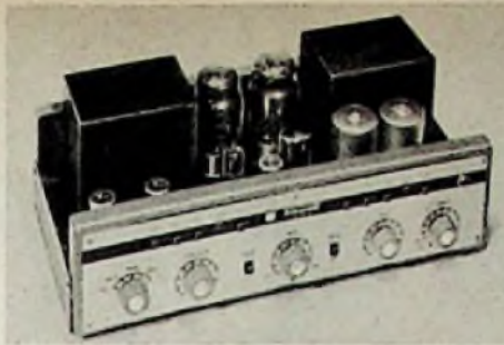
Bild 8. „Telewatt Ultra“, ein 40-W-Hi-Fi-Verstärker (Klein & Hummel)
