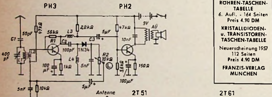
Bild 1. Schaltung des Transistor-Reflexempfängers. Alle Widerstände sind vom 0,5-W-Typ, die Kondensatoren für 10 V Arbeitsspannung
