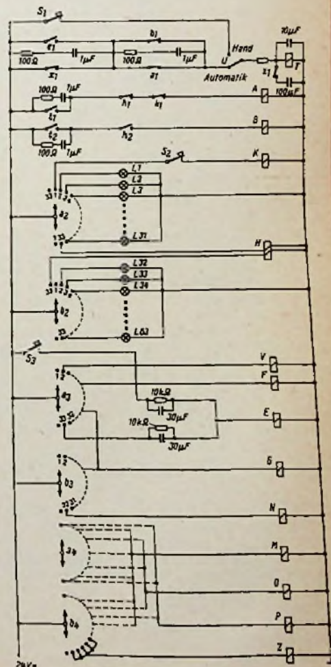
Bild 1. Steuergerät A des Kontrollgerätes für maximal 63 Meßstellen. Die Bezeichnungen sind in allen Zeichnungen einheitlich:
