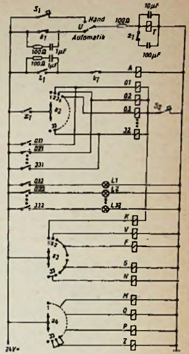
Bild 6. Vereinfachtes Steuerteil B für maximal 32 Meßstellen
