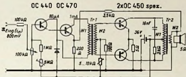
Bild 8. Schaltung eines Niederfrequenzverstärkers mit Intermetall-Siliziumtransistoren für hohe Umgebungstemperaturen.
