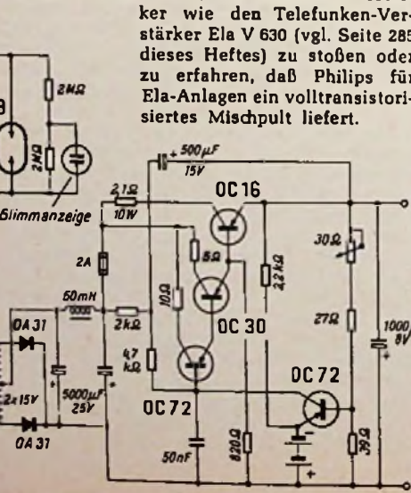
Bild 5. Gleichspannungswandler für 10 W zum Betrieb einer Blützröhre (nach Siemens-Unterlagen)
