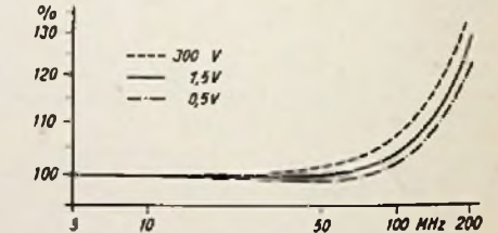
Bild 3. Prozentuale Abweichung der Anzeige des Gerätes als Funktion der Frequenz in MHz bei drei Spannungen
