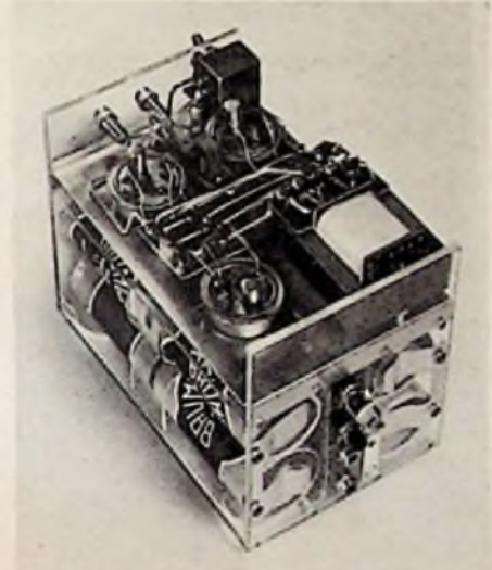
Bild 2. Laborausführung eines Schallplattenverstärkers mit fünf Transistoren von Valvo
