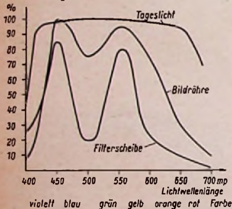
Bild 11. Spektrale Durchlässigkeit der Selektivfilterscheibe im Vergleich zur spektralen Emissionsverteilung der Bildröhre und dem Spektrum des Tageslichtes (Siemens)
