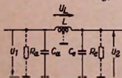
Bild 1. \pi -Schaltung
