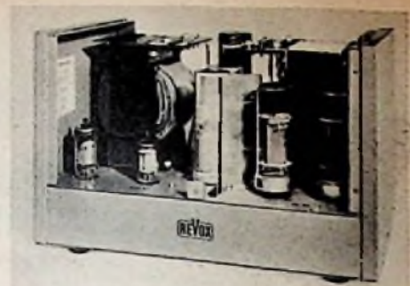
Bild 1. Hi-Fi-Lautsprecherverstärker Revox
