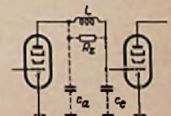
Bild 6. Der zusätzlich bedämpfte \pi -Kreis
