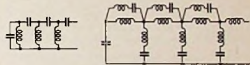
Bild 1. Beliebige Blindwiderstandskombinationen nach dem Wechselwirkungsprinzip
