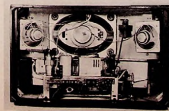
Links: Bild 8. Anordnung der beiden dyn. Hochtonlautsprecher in Telefunken-Operette 6
