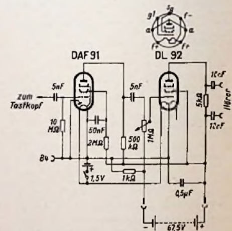
Bild 5. Zweistufiger Signalverfolger
