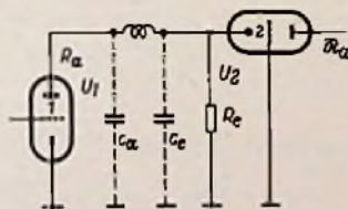
Bild 9. Cascode-Eingangsstufe mit \pi -Glieder als Zwischenkopplung
