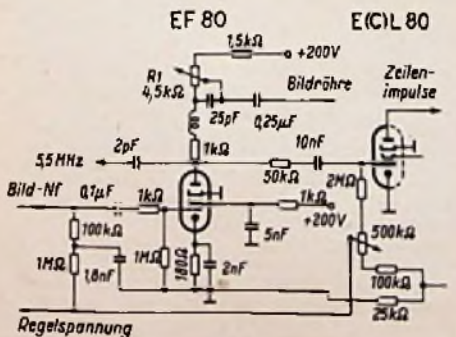
Bild 17. Kontrastregelung und Regelspannungserzeugung in den Krefft-Weltfunk-Empfängern
