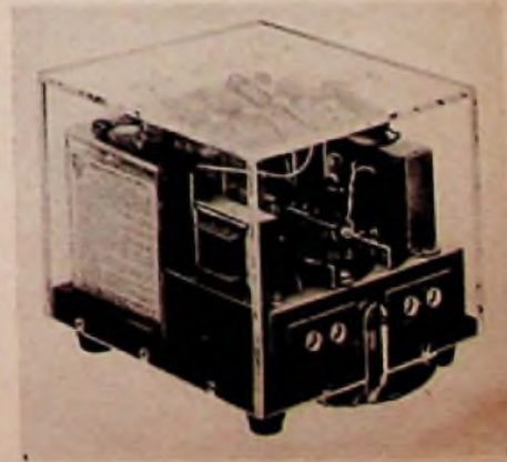
Bild 5. Versuchsausführung eines 5-W-Transistorverstärkers der Firma Graetz
