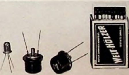
Bild 12. Tekade-Transistoren; links der Vorstufentyp GFT 20, in der Mitte zwei Leistungstransistoren GFT 2006
