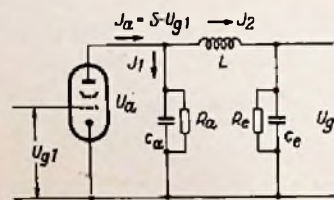
Bild 2. Vierpolersatzschema der \pi -Schaltung
