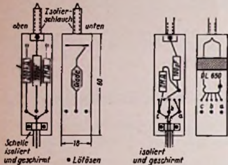
Bild 2. Anordnung der Einzelteile des Tastkopfes mit Germaniumdiode
