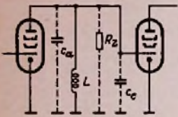
Bild 7. Der zusätzlich bedämpfte Parallelresonanzkreis
