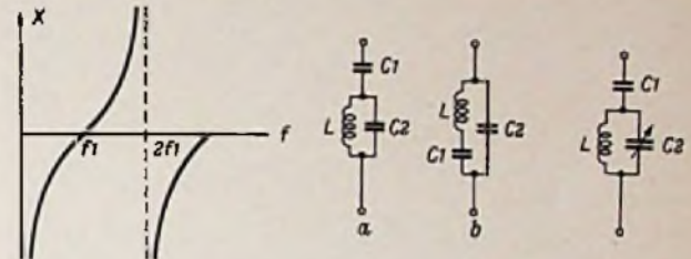
Bild 8. Blindwiderstandsverlauf eines Frequenzverdopplers
