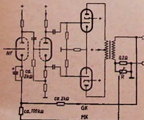
Bild 2. Kombinierte Gegen-Mitkopplung im Verstärker V 120 von Klein & Hummel. G- und M-Kanal sind stark gezeichnet
