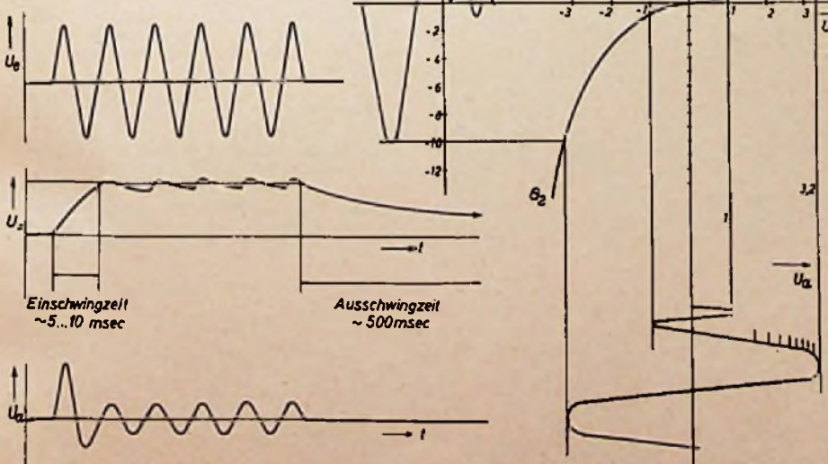
Bild 8. Verlauf der Gleichspannung bei einem Wechselspannungsstoß und dadurch verursachte Ausgangsspannung
