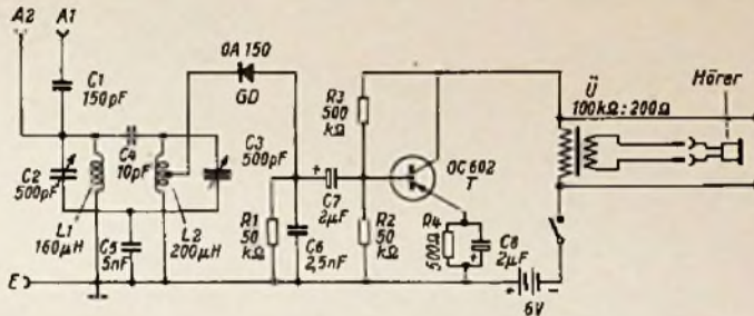
Bild 17. Schaltung des Detektorempfängers mit einstufiger Transistorverstärkung. Durch Vergrößern des Kondensators C4 und Verkleinern des Kondensators C3 läßt sich die Kopplung fester machen
