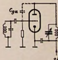
Bild 2. Huth-Kühn-Schaltung
