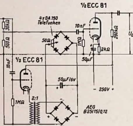
Bild 13. Vollständige Begrenzerschaltung
