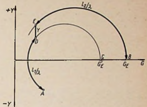
Bild 7. Vergrößerung des Transformationsbereiches durch einen parallel geschalteten Blindwiderstand
