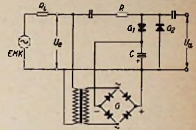
Bild 6. Verbesserte Regelschaltung
