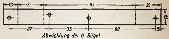
Bild 12. Haltewinkel F, Aluminium 2 mm
