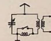
Bild 5. Für kleine Antennen kann die Selbstinduktion des Antennenkreises durch eine Zusatzspule vergrößert werden
