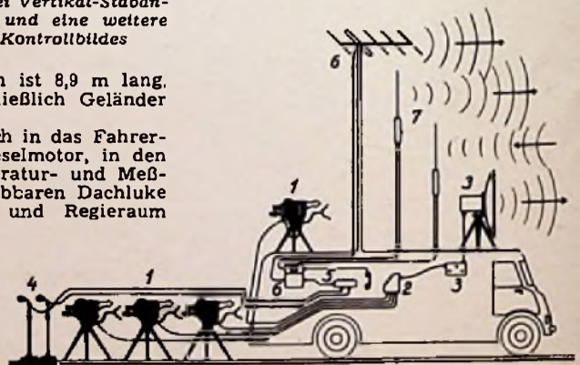
Bild 2. Schema einer Fernseh-Außenübertragung. 1 = Kameras, 2 = Bildmischpult, 3 = Fernseh-Richtfunksender mit Parabol-Strahler, 4 = Mikrofon, 5 = Tonmischpult, 6 = Tonsender, 7 = Gegensprechanlage (Sender und Empfänger)
