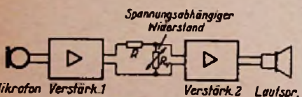
Bild 2. Prinzip einer echten Dynamikregelung
