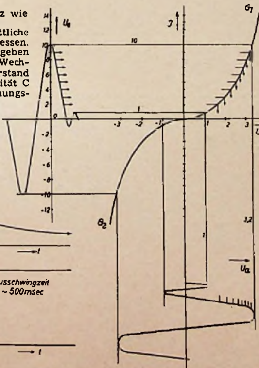
Bild 9. Dynamik-Einengung durch eine Kennlinie nach Bild 5
