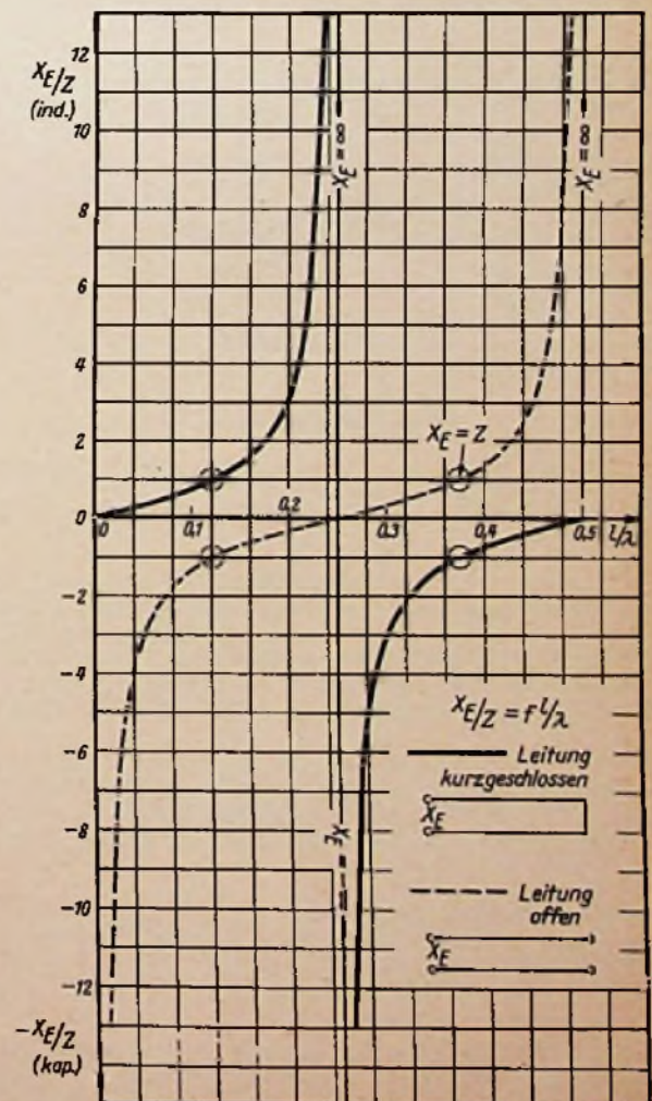
Bild 8. Die Eingangsblindwiderstände von kurzgeschlossenen und offenen Leichterleitungen
