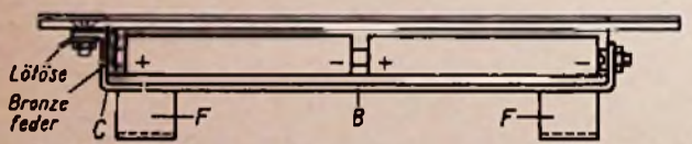
Bild 8. Einteilung der Frontplatte A (Hartpapier 2 mm mit Auflage auf weißem Zellon). B = Metallwinkel für Batterieraum, C = Winkel für Pluspol der Batterien, D = Isolierbrücke zur Verbindung der beiden Batteriewinkel, E = Isolierleiste für Batterieraum, F = zwei Haltewinkel, G = Schiebeshalter
