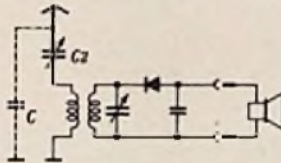
Bild 2. Zweikreis-Detektorempfänger mit Serienschaltung im Antennenkreis
