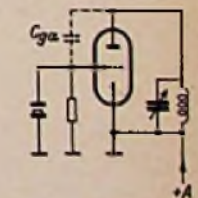
Bild 3. Quarz-Oszillator in Pierce-Miller-Schaltung
