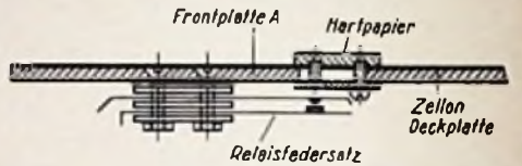
Bild 13. Einzelheiten des Schiebeshalters
