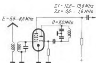
Bild 2. Schaltprinzip des KW-Vorsatzgerätes, betrachtet für das 50-m-Band. Der Eingangskreis ist fest auf Bandmitte (6,2 MHz) abgestimmt
