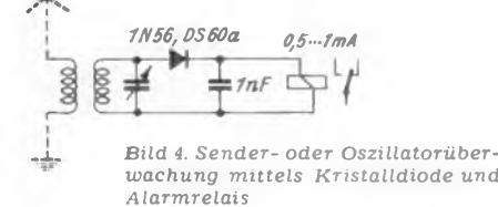
Bild 4. Sender- oder Oszillatorüberwachung mittels Kristalldiode und Alarmrelais
