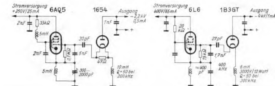
Zwei Beispiele für Röhren-Hochspannungserzeuger mit Serienresonanzkreisen. Beide Schaltungen eignen sich z. B. zur Versorgung kleinerer Katodenstrahloszillografen. Nachbau ist nur nach sorgfältiger Rechnung erfolgversprechend
