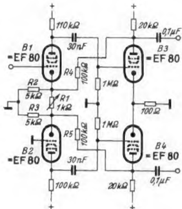
Bild 3. Schaltung des Meßverstärkers
