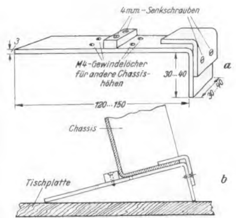
Einfache Chassis-Haltervorrichtung a = Form der Haltewinkel, b = Befestigung am Chassis
