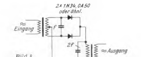
Bild 8. Vollweggleichrichter zur Frequenzverdopplung
