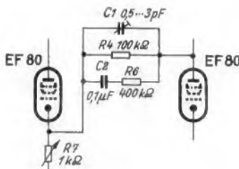
Bild 4. Die Gegenkopplung
