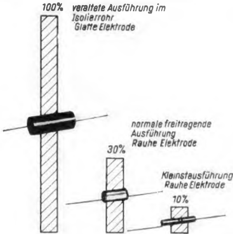
Volumenverminderung bei freitragenden Elektrolyt-Kondensatoren (Siemens)
