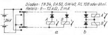
Bild 1. Kristalldioden als stromrichtungsabhängige Schaltglieder in einer Relaischaltung
