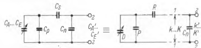
Bild 7. Bandspreizung durch kombinierte Parallel- und Serienkondensatoren zum Drehkondensator
