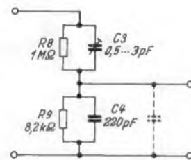
Bild 5. Schaltungsprinzip für die Abschwächer
