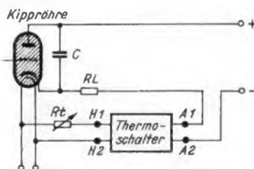
Bild 3. Verwendung des Thermoalters zum Schutz eines Thyratrons
