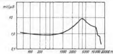
Frequenzkurve des Kristallmikrofons T 44
