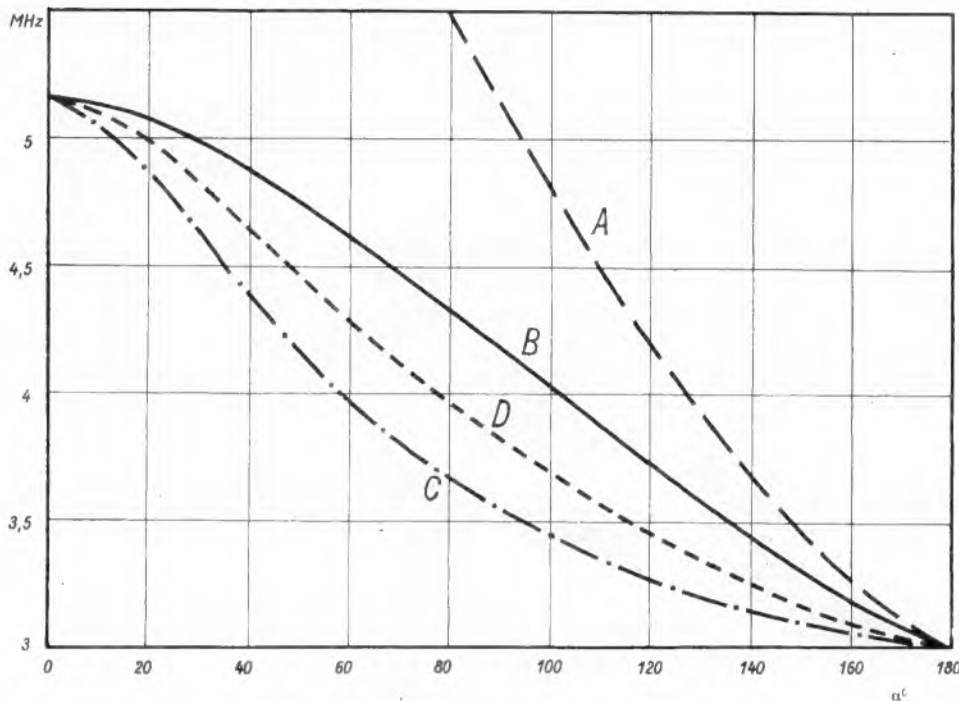
Bild 9. Beispiele zum Skalenverlauf bei verschiedenen Bandspreizmethoden. A nicht gespreizt, B mit Parallel-C-Spreizung, C mit Serien-C-Spreizung, D mit kombinierter Spreizung
