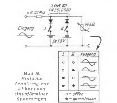
Bild 10. Einfache Schaltung zur Abkappung sinusförmiger Spannungen
