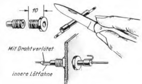
Herstellung von Durchführungskondensatoren aus keramischen Röhrchenkondensatoren
