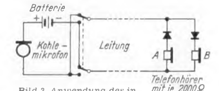
Bild 2. Anwendung des in Bild 1 gezeigten Prinzips auf eine Sprechschaltung
