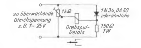
Bild 3. Nichtlineare Brückenschaltung mit Kristalldiode zur Überwachung einer kleinen Gleichspannung
