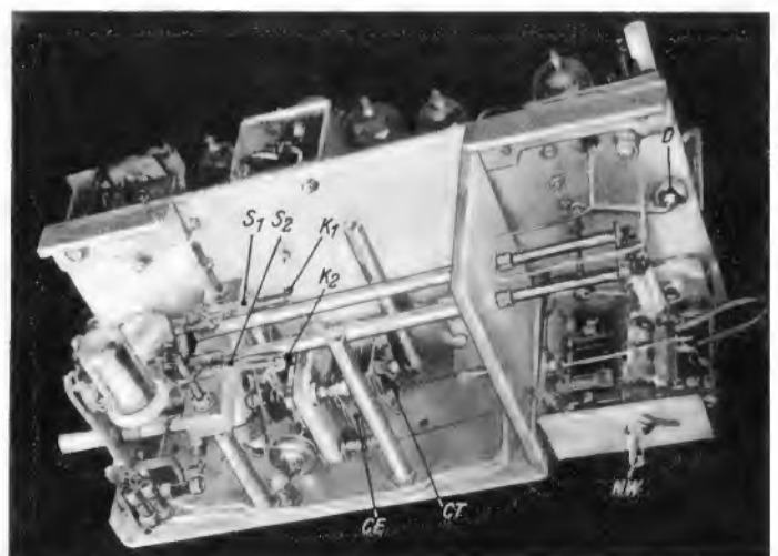
Sender- und Empfängerteil des Hand-Sprechfunk-Gerätes sind übersichtlich aufgebaut. Die Güte der Lecherleitung wird nicht durch zu eng benachbarte Metallteile beeinträchtigt
