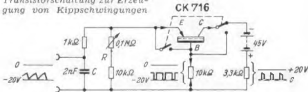
Transistorschaltung zur Erzeugung von Kippschwingungen
