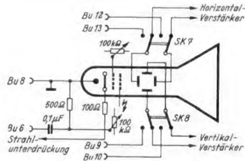
Bild 7. Meßspannungen können auch unmittelbar an die Platten angelegt werden
