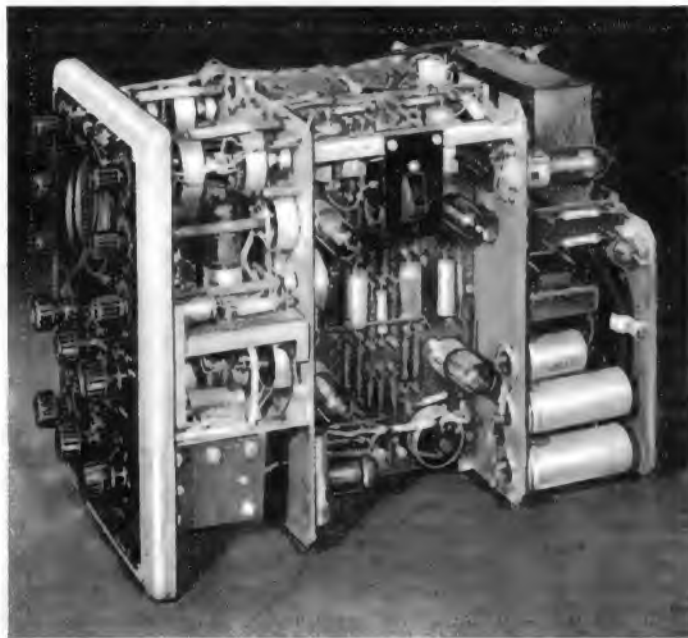
Bild 2. Innenansicht des Elektronenstrahl-Oszillografen GM 5659
