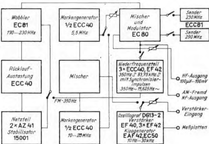
Bild 2. Blockschaltung des Fernseh-Service-Gerätes
