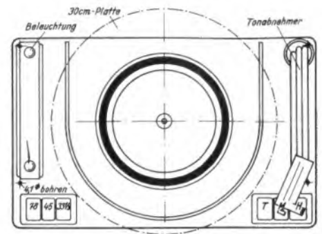
Klaviertasten-Plattenspieler L 103 (Föllner)
