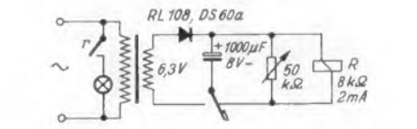
Bild 7. Elektronischer Zeitgeber mit Kristalldiode, z. B. für ein Fotokopiergerät
