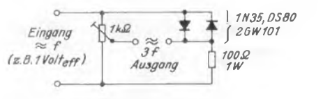
Bild 9. Frequenzverdreifachung in einer nichtlinearen Brückenschaltung
