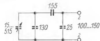
Bild 8. Schaltung zum Beispiel zu Verfahren D mit errechneten Werten für C_p und C_s
