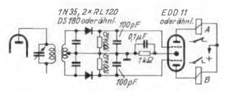
Bild 6. Schaltung zur Überwachung der Frequenz eines Senders
