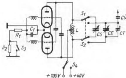
Gegentaktoszillator des Hand-Sprechfunk-Gerätes. Stellung S_1 = Sender-Oszillator, S_2 = Empfangs-Oszillator
