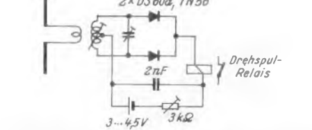
Bild 5. Einfache Empfangsschaltung für drahtlose Fernsteuerung im 144 MHz-Band
