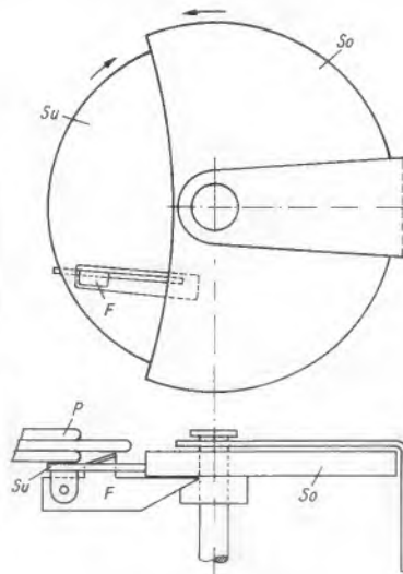
Bild 6. Dual-Fühlhebelsmechanismus
