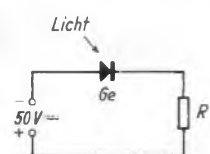
Bild 4. Schaltung der Fotodiode 1 N 77
