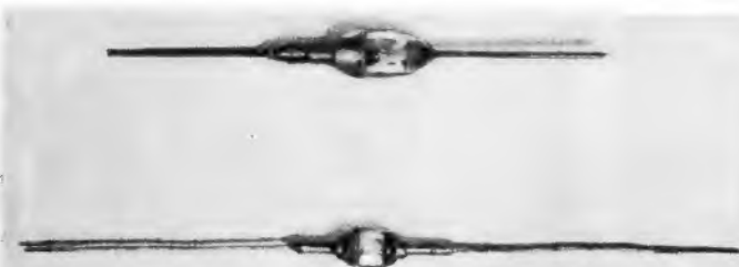
Bild 1. Oben: Glasdiode, Ausführung Bull 1942; unten: Glasdiode 1 N...A 1951
