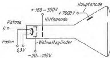
Bild 62. Grundsätzliche Elektrodenanordnung bei normalen Bildröhren
