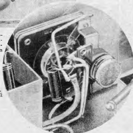
Oben: Bei abgenommener Abschirmhaube sehen wir deutlich die Anordnung der Einzelteile in den drei oberen Kammern.
