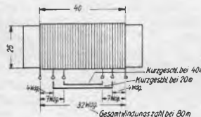
Die Sender-spule mit ihren Abmessungen und den Anzapfungen für den Wellen-schalter.
