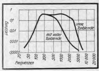
Die Tonblende setzt die Lautstärke der hohen Töne erheblich herab.
