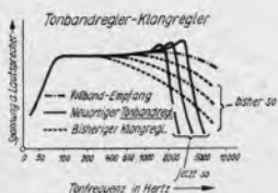
Abb. 1. Die Wirkungsweise des Tonbandreglers gegenüber der einer üblichen Tonblende.
