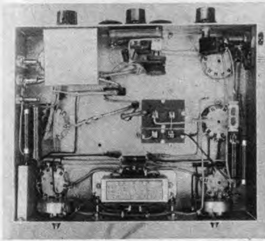
Die Verdrahtung macht wenig Mühe, weil wenig Leitungen zu ziehen sind und genügend Platz vorhanden ist.
