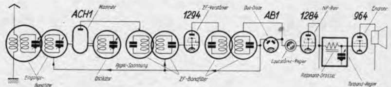
Abb. 2. Das Schaltbild eines Vorröhren-Supers. Vor dem Gitter der Endröhre der Tonbandregler.
