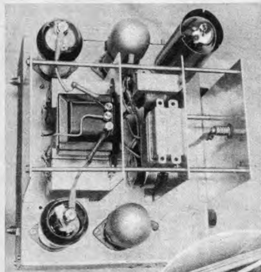
Oben: Bei abgenommener Abschirmhaube sehen wir deutlich die Anordnung der Einzelteile in den drei oberen Kammern.
