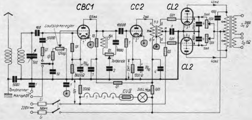
Das Schaltbild des Gleichstromverstärkers. Der Verstärker hat einen eingebauten Abstimmkreis, so daß Rundfunkwiedergabe möglich ist. Der Lautstärkeregel befindet sich vor der ersten Röhre, der Klangregler vor der zweiten.
