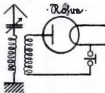
Abb. 1. Die Detektorwirkung der Röhre: Der Strom kann nur in der einen Richtung durch, in der anderen findet er einen unendlich hohen Widerstand vor.
