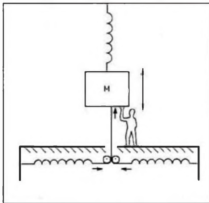
Fig. 8 Simil mecánico de la resonancia de una vertical con radiales
