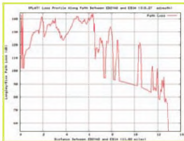
Figura 3. Atenuación entre EB1A y ED2YAD según SPLAT! en función de la distancia desde EB1A (ver texto).
