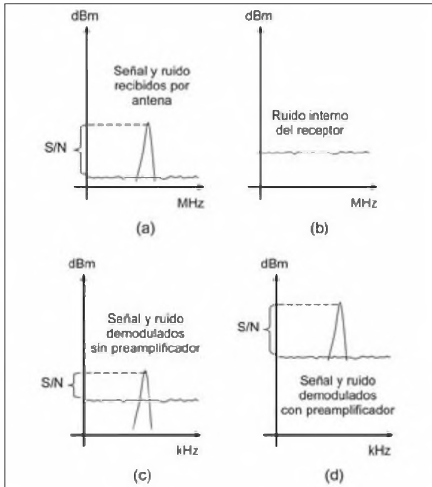
Figura 1. Se describe una situación típica de VHF y bandas superiores: señal débil y ruido entrante por antena inferior al ruido interno del receptor: ver texto acerca de la utilidad de un preamplificador de recepción en casos como éste.
