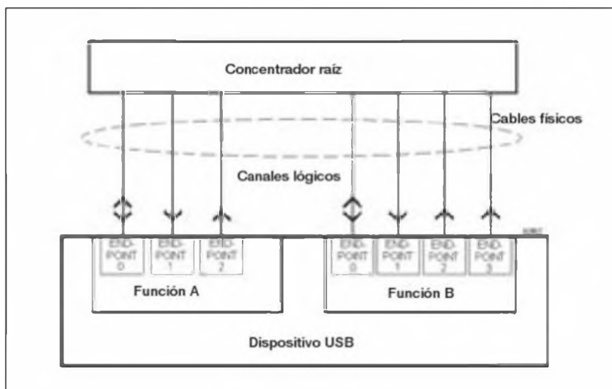
Figura 1. Este esquema te ayudará a comprender la relación entre la conexión USB y el concentrador raíz , las diferentes partes del dispositivo y los canales lógicos que transportan los datos. Todas estas conexiones lógicas son como si fueran una conexión física por cable.
