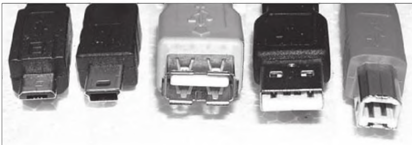
Figura 3. Varios conectores USB: Micro-A, Mini-B, Hembra tipo A, Macho tipo A, y conector tipo B. Observa los dos contactos exteriores del conector macho tipo A, son un poco más largos que los de datos, de modo que se conecten primero.
