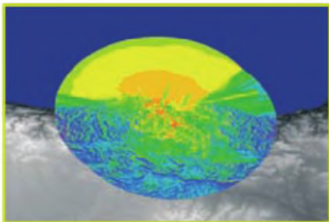
Foto I. Mapa de cobertura conjunta de EB1A y ED2YAD, suponiendo que operasen en la misma frecuencia.
