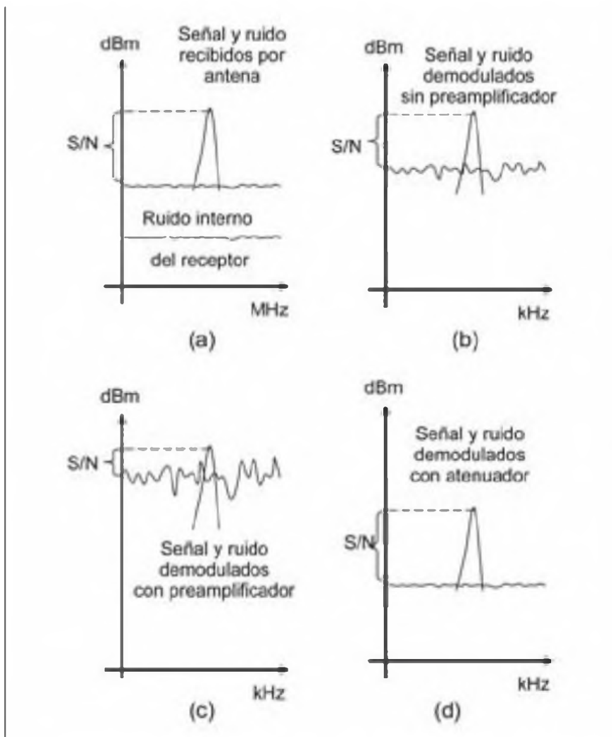
Figura 2. Se muestra el caso típico de recepción en HF, donde el ruido externo captado por la antena es muy superior al ruido interno del receptor. Si en esta situación activamos el preamplificador, se corre el riesgo de estropear la relación S/N, haciendo que en (c) la señal quede enmascarada por el ruido. En cambio, en (d), insertando el atenuador en la entrada descienden tanto la señal como el ruido exterior, pero manteniendo la relación S/N original.
