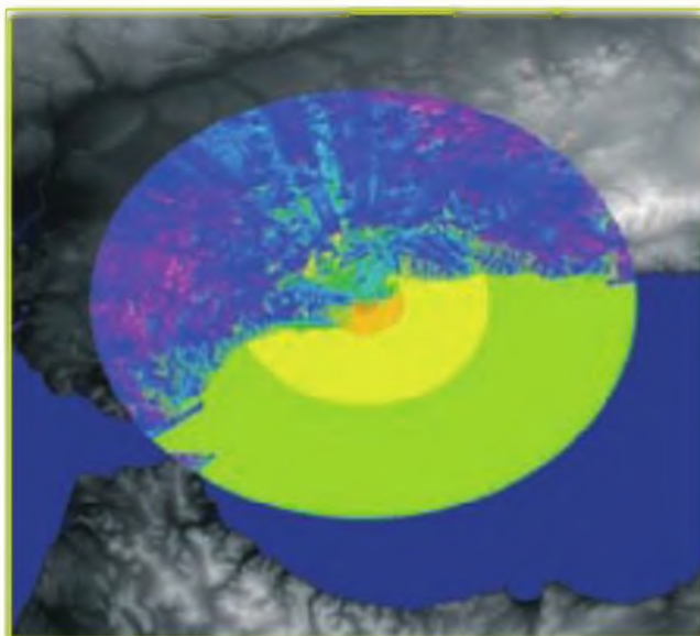
Fotos E, F y G. Cobertura según SPLAT! desde el Cerro del Moro en las bandas de 50, 145 y 432 MHz respectivamente. Cuanto más vivo es el color en un área, mejor las señales (ver texto).
