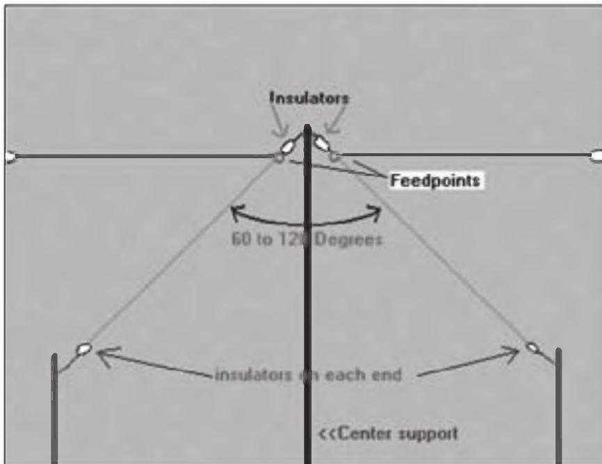
Esta ilustración muestra una antena en V invertida (cables naranja). Los cables azules muestran una configuración horizontal, en la que los extremos están a la misma altura que el centro de la antena.
