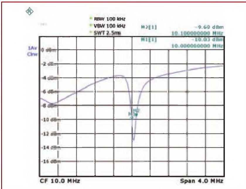
Gráfico. Respuesta de la YP-3 de Super antenna en 30 metros.
