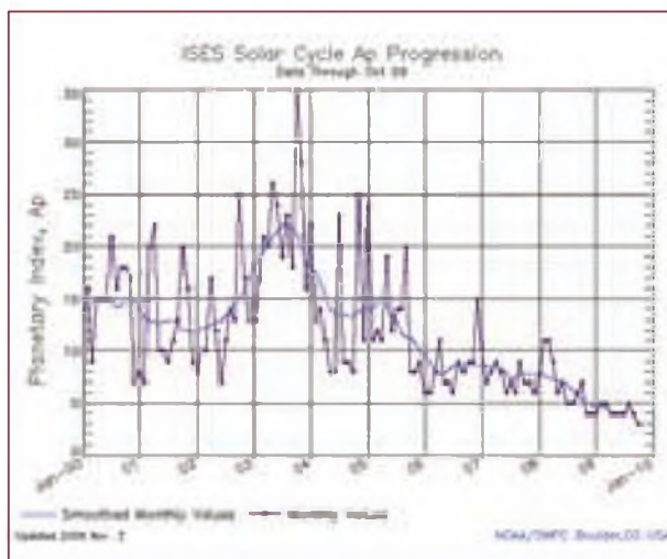
Figura 3. Los valores del índice planetario Ap, que mostraban notables variaciones hasta el año 2006, han moderado sus oscilaciones y tienden, aparentemente, hacia una temporada de baja actividad. (Cortesía NOAA)
