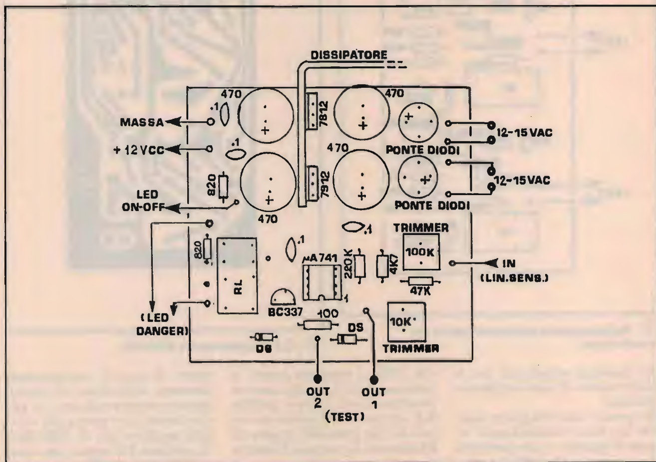
⑥ Posizionamento componenti sul C.S. dell'alimentatore duale e amplificatore di segnale del sensore.
