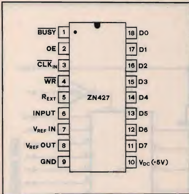
⑤ Connessioni dei circuiti integrati utilizzati e relative funzioni.
