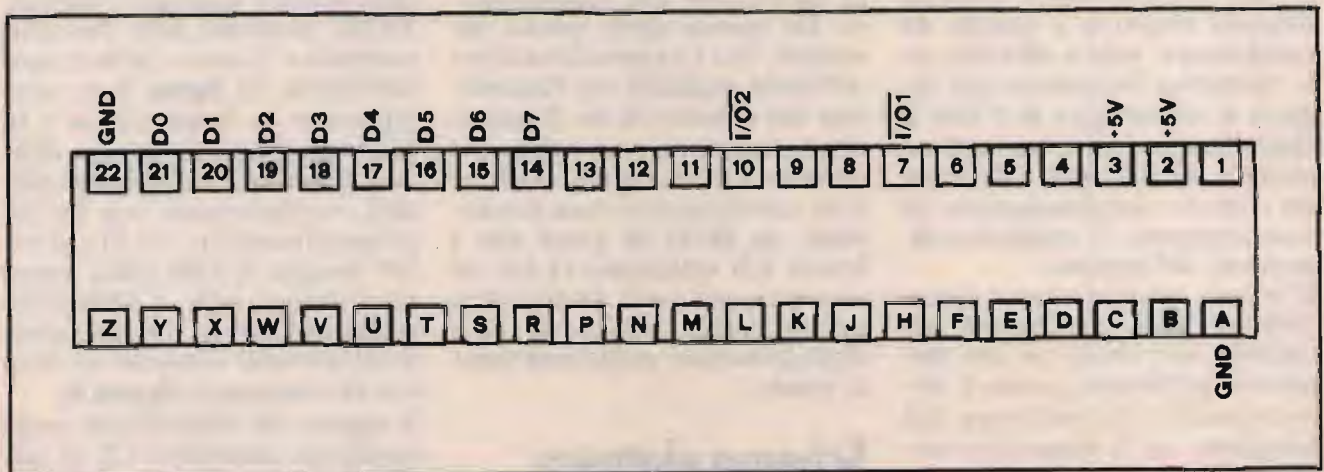
⑥ Connessioni e relative funzioni della EXPANSION PORT del C64 (vista frontale).
