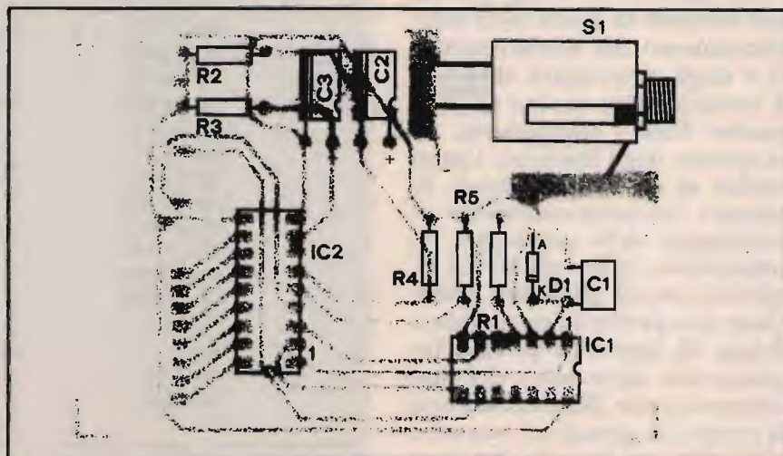
4 Disposizione dei componenti sul circuito stampato.
