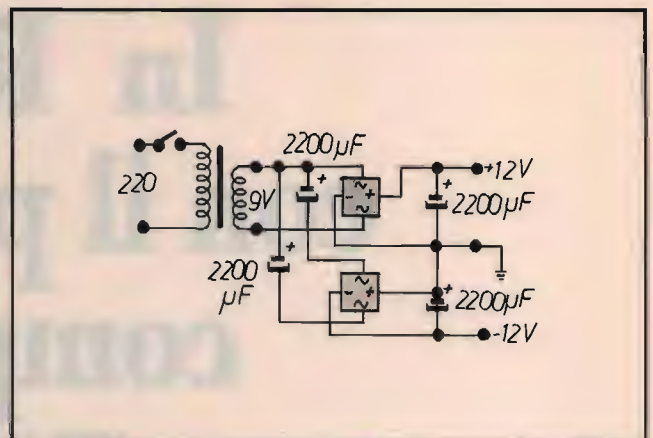
③ Alimentatore duale.
