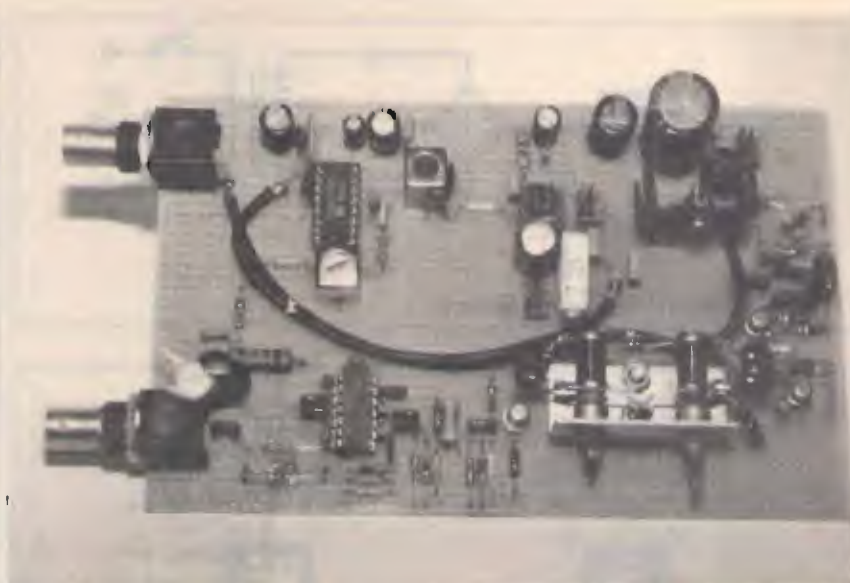
foto 2 Ricevitore ultimato.
