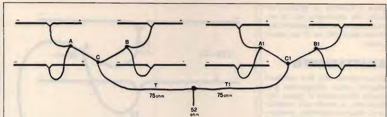
figura 6 Connessione in parallelo di otto antenne sovrapposte a due a due e collegate in due gruppi di quattro.
