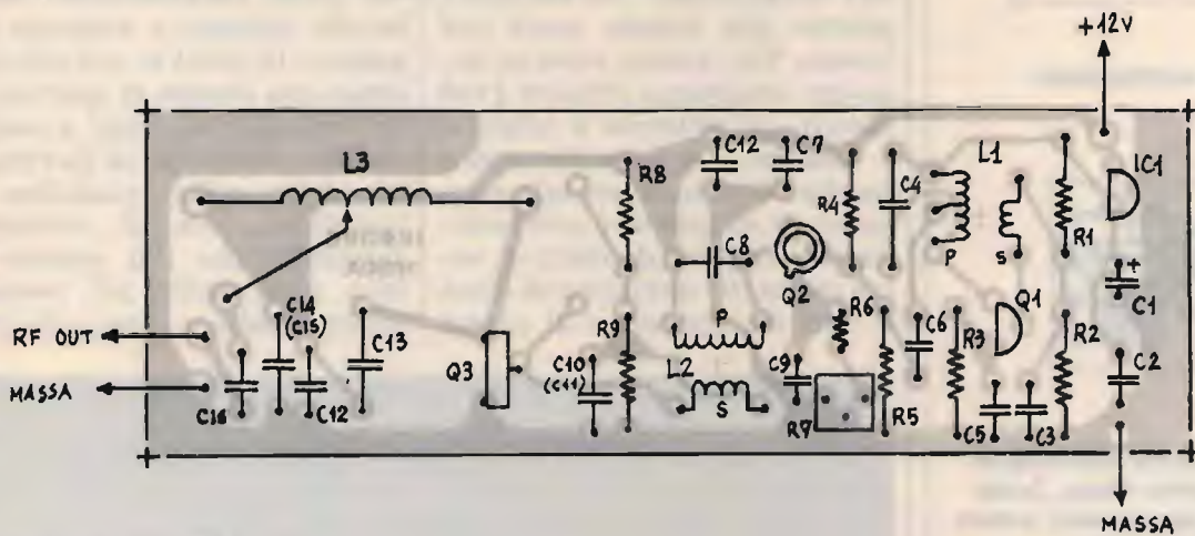
Disposizione componenti.
