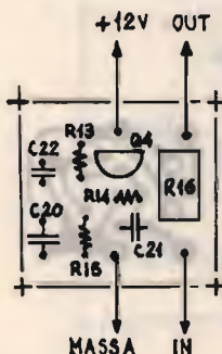
Disposizione componenti.
