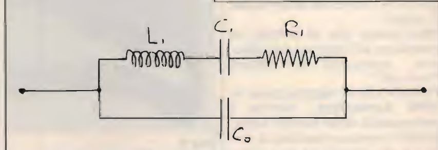
Distribuzione RLC semplificata in un cristallo di quarzo.
