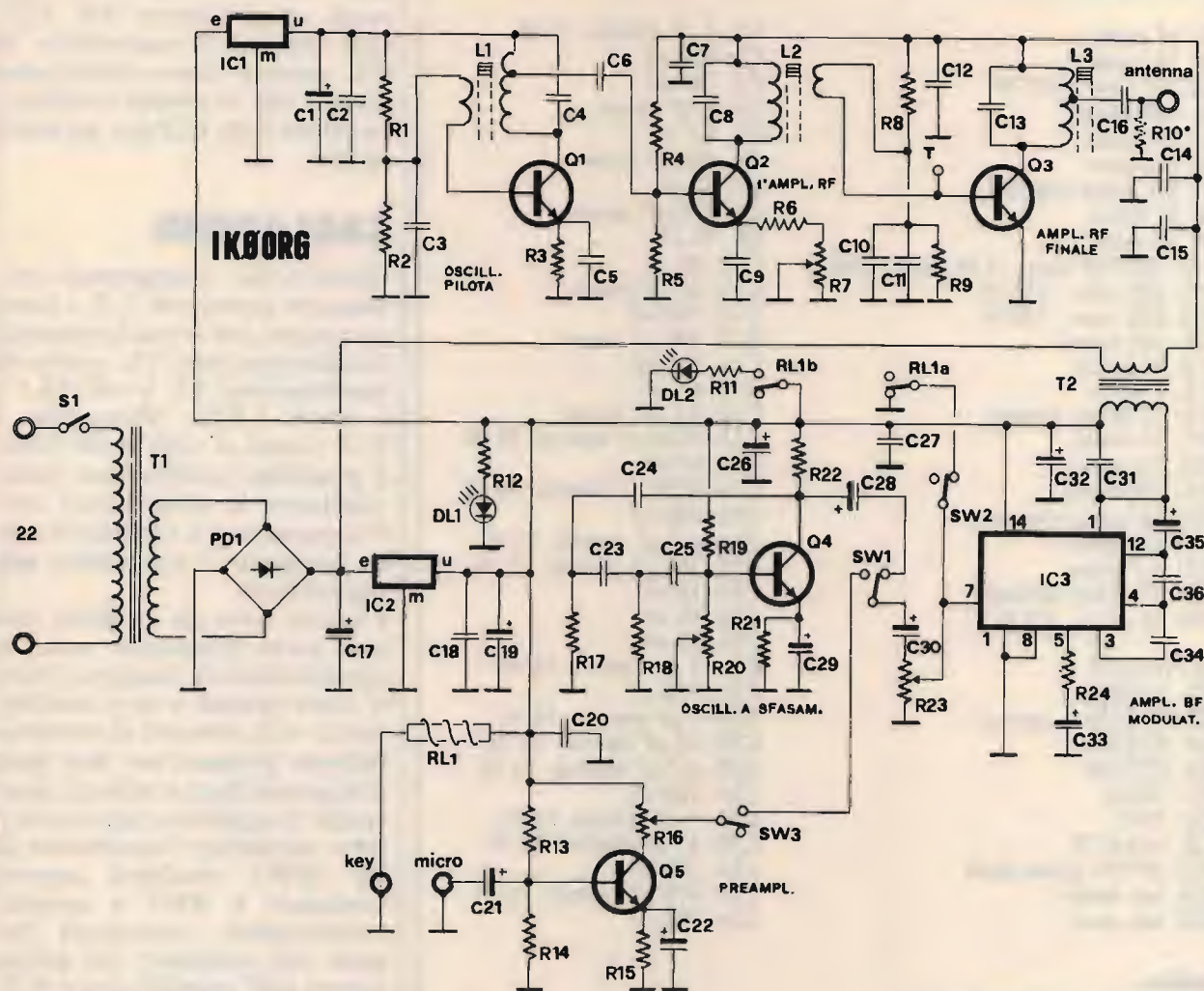
Schema elettrico.
