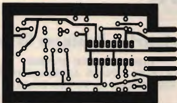
figura 2 Disegno del circuito stampato.
