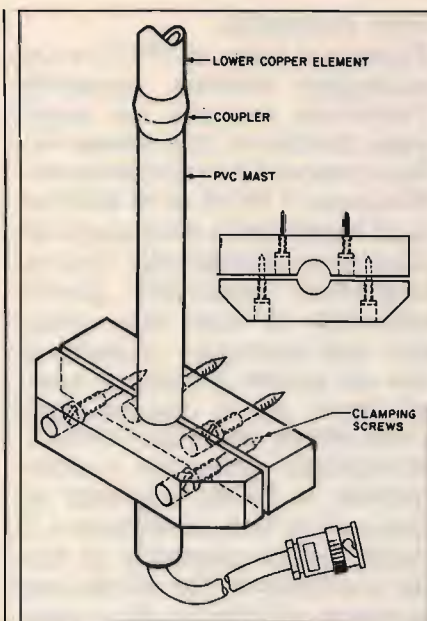
figura 2 Dettaglio del sistema di montaggio. Lower copper element = tubo metallico inferiore; coupler = giunto; PVC mast = palo in PVC; clamping screws = viti di fissaggio.
