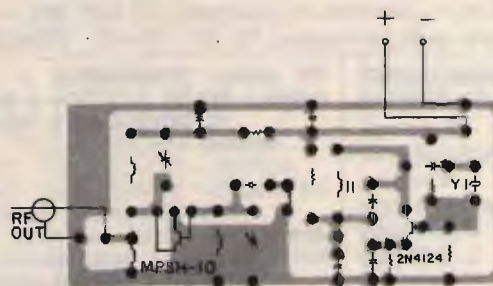
figura 3 Schema pratico di montaggio.
