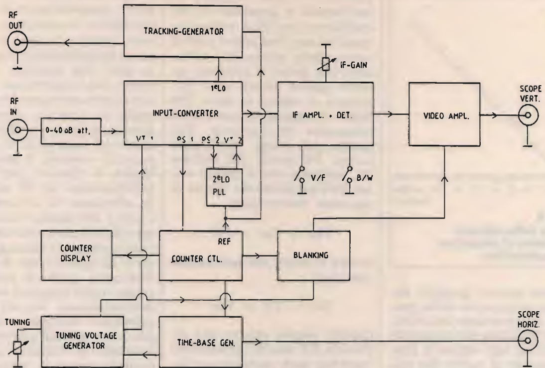
figura 1 Schema a blocchi dello Spectrum Analyzer HM 8028.
