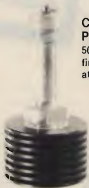
TRASFORMATORE COASSIALE DI IMPEDENZA 50 ohm - 75 ohm attacco C L. 30.000
