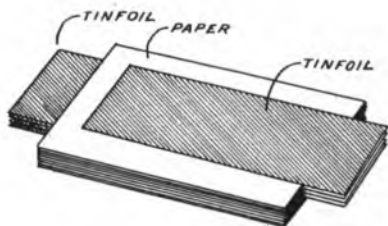
FIG. 80.—Fixed condenser.
