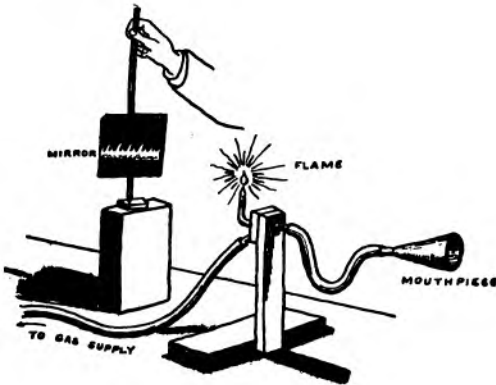
FIG. 129.—Koenig's manometric flame apparatus.
