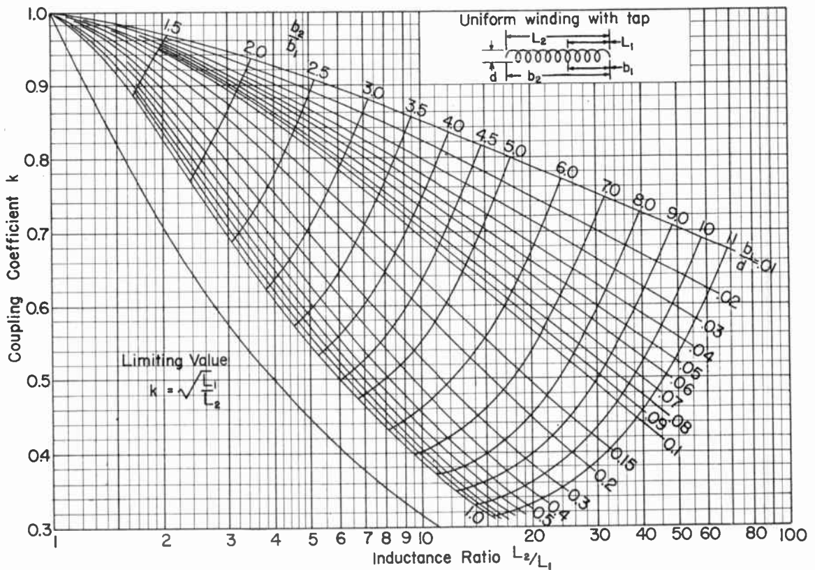
Fig. 3—Auto transformer.
