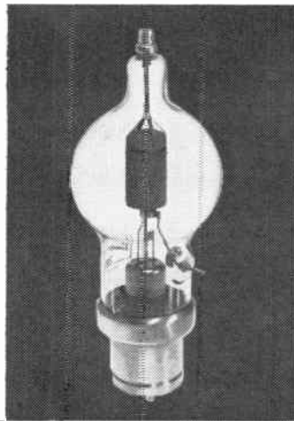
250w Triode
