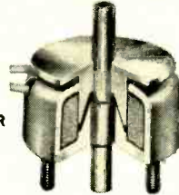
LEDEX CONICAL PLUNGER (Medium Stroke)
