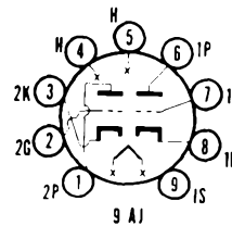
SYLVANIA TYPE 6BZ7 VHF DUO TRIODE
