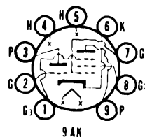
SYLVANIA TYPE 6X8 H F TRIODE PENTODE
