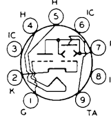
6DA5
