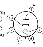
6W4-GT
