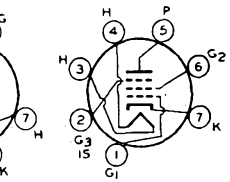
12EA6
