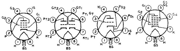
14A7 14A7/12B7 14AF7 14B6 14B8
