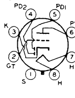
6ST7
