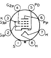
6SV7
