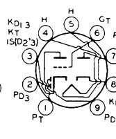
6V8
