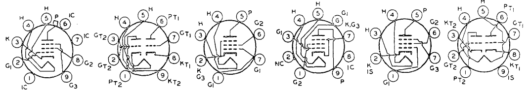
6DT8
