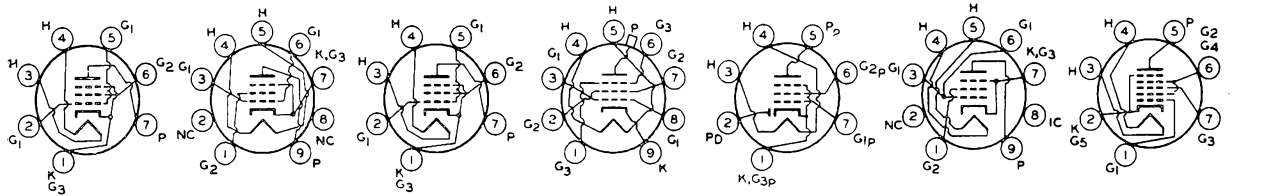
12CM6
