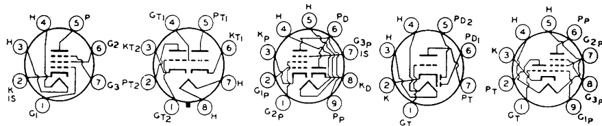
6AS6
