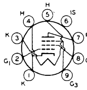
6BX6
