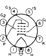
12B7
