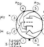
12SQ7-GT 12SR7-GT 12SW7
