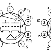
6BQ7 6BQ7-A
