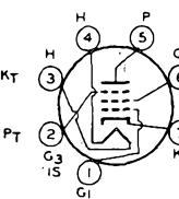
12DZ6
