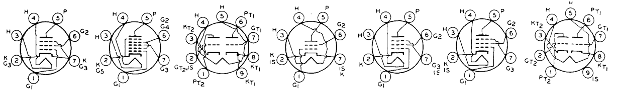
4CE5
