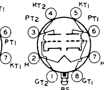
7F8
