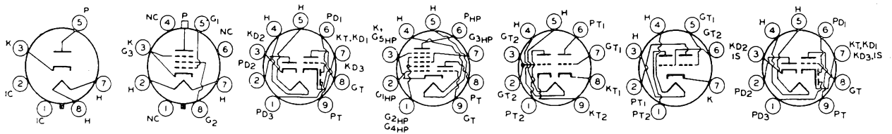
19D8
