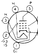
26CG6
