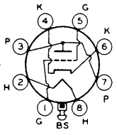
7E5
