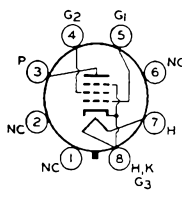
6V5-GT
