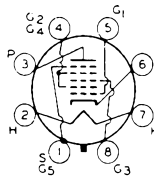
12SA7
