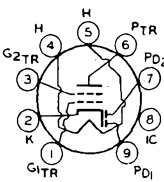
12DU7
