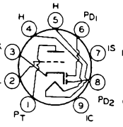
6BD7
