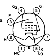
12EF6
