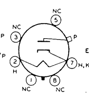
6Y3-G
