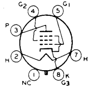
6Y6-G 6Y6-GA 6Y6-GT
