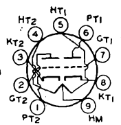
12DT7
