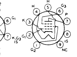
6CK6
