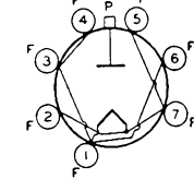
1Z2
