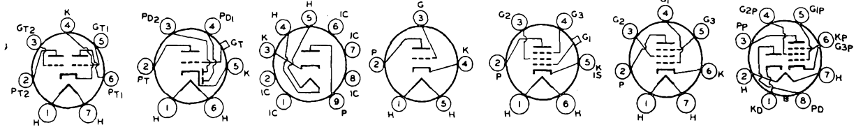
70L7-GT
