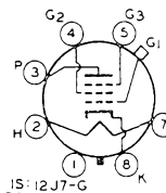
12J7-G 12J7-GT
