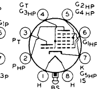
7S7
