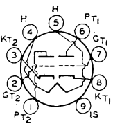
12DT8
