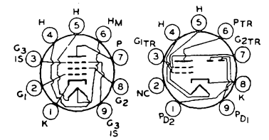
12DS7
