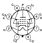
6CL5
