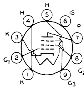
6BY7
