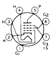
6DE6
