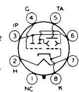
6DL7
