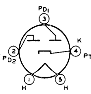
84/6Z4
