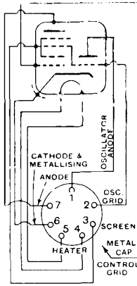
TRIODE-HEXODES
