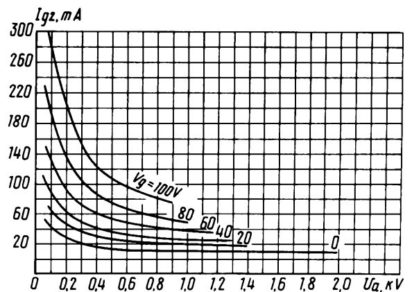
Усредненные сеточно-анодные характеристики (по сетке второй): U_i = 10 \text{ В}; U_{g2} = 0.4 \text{ кВ}; напряжение лучеобразующих пластин ( U_{пн} ) равно 0 В Averaged Grid 2-Anode Characteristic Curves: U_i = 10 \text{ V}; U_{g2} = 0.4 \text{ kV}; beam-forming plates voltage U_{пн} is 0
