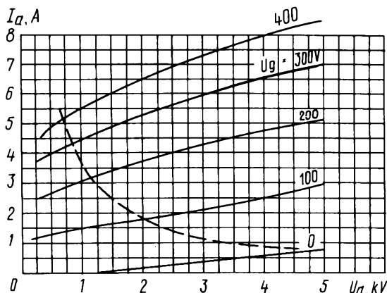
Усредненные анодные характеристики: U_i = 12,6 \text{ В} ; - - - - - наибольшая мощность, рассеиваемая анодом ( P_{a, \text{max}} ) Averaged Anode Characteristic Curve: U_i = 12,6 \text{ V} ; - - - - - P_{a, \text{max}}
