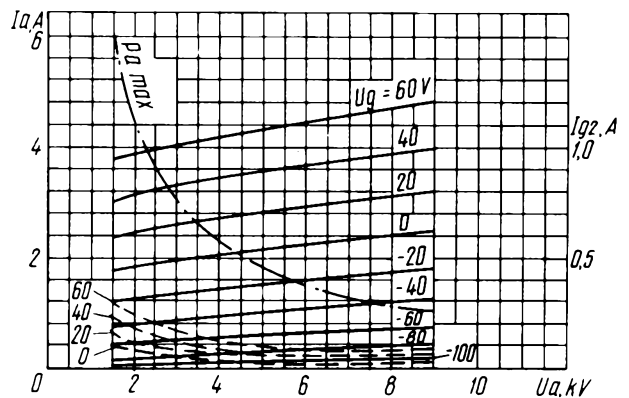
Усредненные характеристики: U_f = 5 \text{ В} ; U_{g2} = 1 \text{ кВ} ; ——— анодные; - - - - сеточно-анодные; - · - · наибольшая мощность, рассеиваемая анодом ( P_{a \text{ max}} ) Averaged Characteristic Curves: U_f = 5 \text{ В} ; U_{g2} = 1 \text{ кВ} ; ——— anode; - - - - grid-anode; - · - · P_{a \text{ max}}
