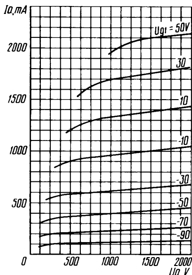
Усредненные анодные характеристики: U_i = 8,3 В; U_{g2} = 0,6 кВ; U_{g3} = 0 В Averaged Anode Characteristic Curves: U_i = 8.3 V; U_{g2} = 0.6 kV; U_{g3} = 0 V
