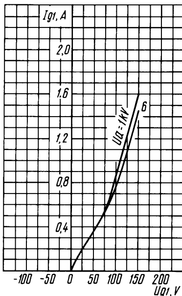
Усредненные сеточные характеристики (по сетке первой): U_1 = 8.3 \text{ В}; U_{q2} = 1.2 \text{ кВ} Averaged Grid 1 Characteristic Curves: U_1 = 8.3 \text{ V}; U_{q2} = 1.2 \text{ кВ}
