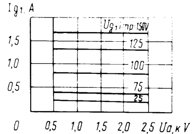
Усредненные импульсные сеточно-анодные характеристики (по сетке второй): U_1 = 12,6 В; U_{g2} = 800 В
