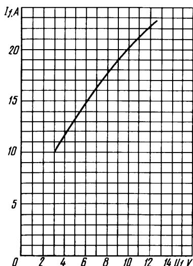
Усредненная накальная характеристика (сопротивление накального катода составляет около 0,06 Ом)
