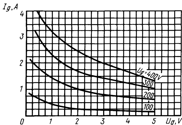
Усредненные сеточно-анодные характеристики: U_i = 12,6 В
