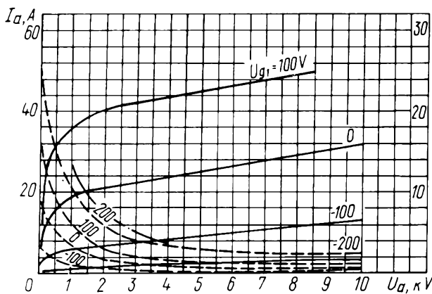
Усредненные характеристики: U_f = 14 \text{ В}; U_{g2} = 1,5 \text{ кВ}; ——— анодные; - - - - - сеточно-анодные; - · - · - · наибольшая допустимая мощность, рассеиваемая анодом ( P_{a \text{ max}} )
