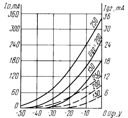
Усредненные характеристики: U_i = 12,6 V; U_a = 800 V; U_{g3} = 0 V ——— анодно-сеточные; - - - - сеточные (по сетке второй) Averaged Characteristic Curves: U_i = 12.6 V; U_a = 800 V; U_{g3} = 0 ——— anode-grid; - - - - grid 2
