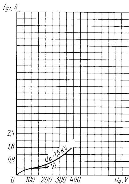
Усредненные сеточные характеристики (по сетке второй): U_i = 6,3 \text{ В}; U_{g2} = 1,5 \text{ кВ} Averaged Grid 2 Characteristic Curves: U_i = 6.3 \text{ V}; U_{g2} = 1.5 \text{ kV}
