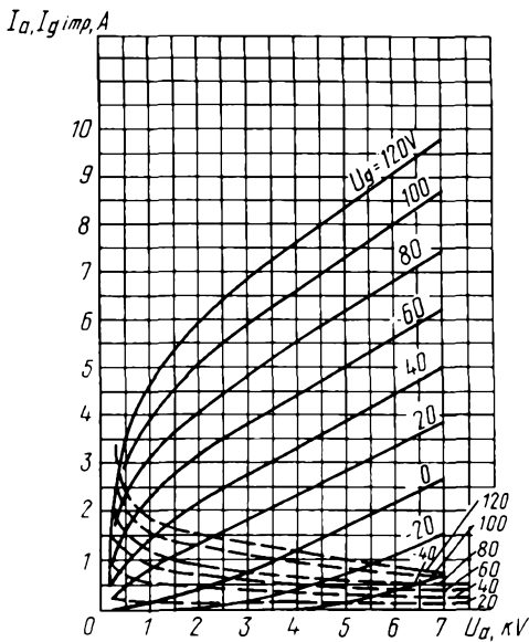
Усредненные импульсные характеристики: U_f = 12,6 В; \tau_{imp} = 4 мкс; частота посылок ( f_p ) равна 350 имп/с; ——— анодные; - - - - сеточно-анодные Averaged Pulse-Operation Characteristic Curves: U_f = 12,6 V; \tau_{imp} = 4 \mu s; frequency 350 imp/s; ——— anode; - - - - grid-anode
