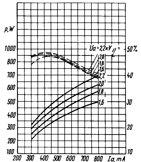
Усредненные характеристики зависимости полезной мощности и коэффициента полезного действия от тока анода: U_i = 12,6 В; \lambda = 30 см; — полезная мощность (P); - - - коэффициент полезного действия ( \eta ) Averaged Characteristic Curves Showing Output Power and Efficiency versus Anode Current: U_i = 12.6 V; \lambda = 30 cm; — output power (P); - - - efficiency ( \eta )
