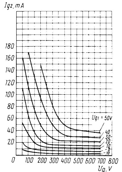
Усредненные сеточно-анодные характеристики (для одного тетрода): U_i = 6,3 \text{ В}; U_{g2} = 200 \text{ В} Averaged Grid-Anode Characteristic Curves (Each Tetraode): U_i = 6.3 \text{ V}; U_{g2} = 200 \text{ V}
