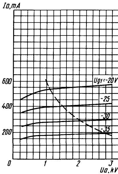
Усредненные анодные характеристики: U_i = 12,6 \text{ В}; U_{g2} = 250 \text{ В}; - - - - - наибольшая мощность, рассеиваемая анодом ( P_{a,max} )
