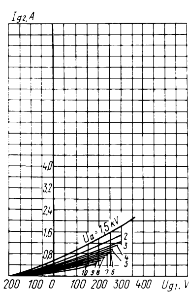
Усредненные сеточные характеристики (по сетке второй): U_i = 6,3 \text{ В}; U_{g2} = 1,5 \text{ кВ} Averaged Grid 2 Characteristic Curves: U_i = 6.3 \text{ V}; U_{g2} = 1.5 \text{ kV}
