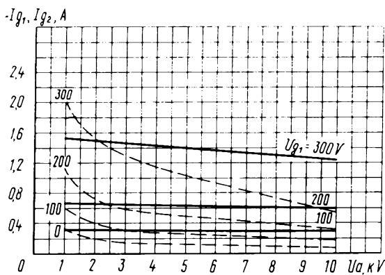
Усредненные характеристики: U_i = 6,3 \text{ В}; U_{g2} = 1 \text{ кВ}; — сеточно-анодные (по сетке первой); - - - сеточно-анодные (по сетке второй) Averaged Characteristic Curves: U_i = 6.3 \text{ V}; U_{g2} = 1 \text{ kV}; — grid 1-anode; - - - grid 2-anode
