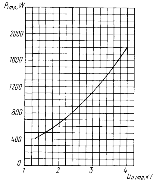
Усредненные импульсные характеристики: U_f = 12,6 В; \tau_{imp} = 4 мкс; частота посылок ( f_p ) равна 350 имп/с; ——— анодные; - - - - сеточно-анодные Averaged Pulse-Operation Characteristic Curves: U_f = 12,6 V; \tau_{imp} = 4 \mu s; frequency 350 imp/s; ——— anode; - - - - grid-anode
