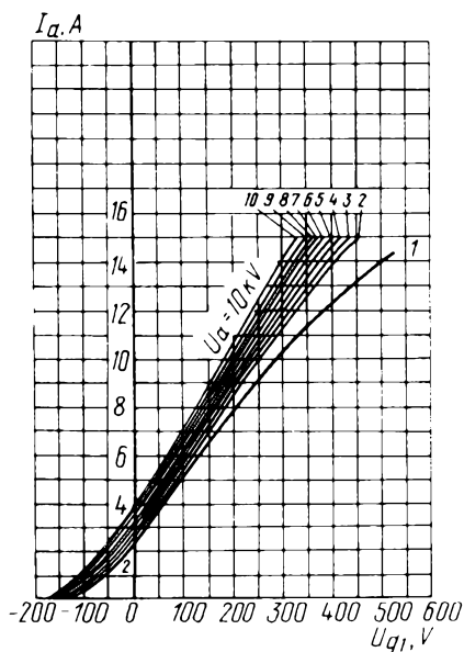
Усредненные анодно-сеточные характеристики: U_i = 6,3 \text{ В}; U_{g2} = 1,5 \text{ кВ} Averaged Anode-Grid Characteristic Curves: U_i = 6.3 \text{ V}; U_{g2} = 1.5 \text{ kV}
