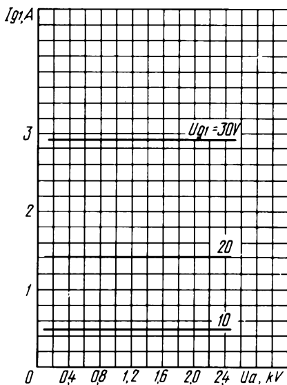
Усредненные сеточно-анодные характеристики:
