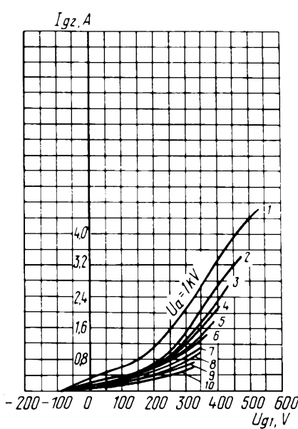
Усредненные сеточные характеристики (по сетке второй): U_i = 6,3 \text{ В}; U_{g2} = 1 \text{ кВ} Averaged Grid 2 Characteristic Curves: U_i = 6.3 \text{ V}; U_{g2} = 1 \text{ kV}
