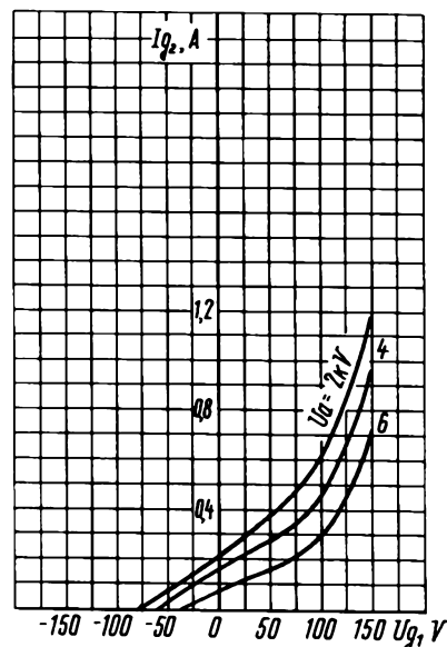
Усредненные сеточные характеристики (по сетке второй): U_1 = 8.3 \text{ В}; U_{q2} = 1.2 \text{ кВ} Averaged Grid 2 Characteristic Curves: U_1 = 8.3 \text{ V}; U_{q2} = 1.2 \text{ кВ}
