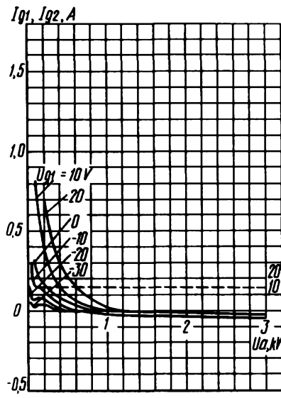
Усредненные характеристики: U_i = 12,6 \text{ В}; U_{g2} = 250 \text{ В}; — сеточно-анодные (по сетке второй); - - - - - сеточно-анодные (по сетке первой)
