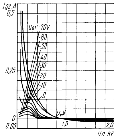
Усредненные сеточно-анодные характеристики (по второй сетке): U_i = 12,6 В; U_{g2} = 350 В
