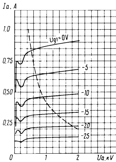
Усредненные анодные характеристики: U_i = 6,3 \text{ В}; U_{g2} = 300 \text{ В}; ——— ток анода ( I_a ); - - - - наибольшая мощность, рассеиваемая анодом ( P_{a \text{ max}} ) Averaged Anode Characteristic Curves: U_i = 6.3 \text{ V}; U_{g2} = 300 \text{ V}; ——— I_a ; - - - - P_{a \text{ max}}
