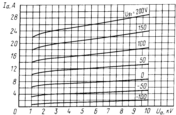
Усредненные анодные характеристики: U_f = 8,3 \text{ В}; U_{g2} = 1 \text{ кВ} Averaged Anode Characteristic Curves: U_f = 8.3 \text{ В}; U_{g2} = 1 \text{ кВ}
