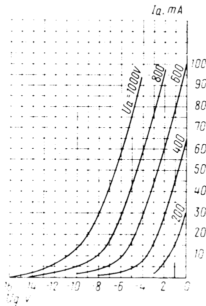
Усредненные анодно-сеточные характеристики: U_i = 12,6 \text{ В}
