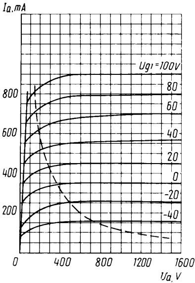
Усредненные анодные характеристики: — — — — — наибольшая мощность, рассеиваемая анодом ( P_{a,max} ); U_1 = 20 В; U_{g2} = 0,4 кВ; U_{g3} = 50 В Averaged Anode Characteristics: U_1 = 20 V; U_{g2} = 0.4 kV; U_{g3} = 50 V; - - - - - P_{a,max}
