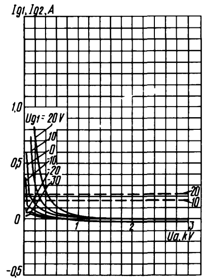
Усредненные характеристики: U_i = 12,6 \text{ В}; U_{g2} = 300 \text{ В}; — сеточно-анодные (по сетке второй); - - - - - сеточно-анодные (по сетке первой)
