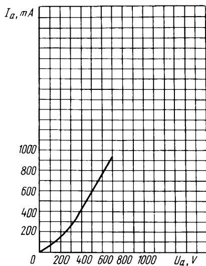
Усредненная анодная характеристика: U_i = 6,3 В Averaged Anode Characteristic Curve: U_i = 6.3 V
