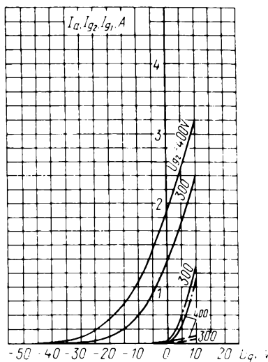
Усредненные характеристики: U_1 = 12,6 \text{ В}; U_a = 100 \text{ В}; — — — — — анодно-сеточные; - - - - - сеточные (по сетке второй); - - - - - сеточные (по сетке первой) Averaged Characteristic Curves: U_1 = 12.6 \text{ V}; U_a = 1,000 \text{ V}; — — — — — anode-grid; - - - - - grid 2; - - - - - grid 1
