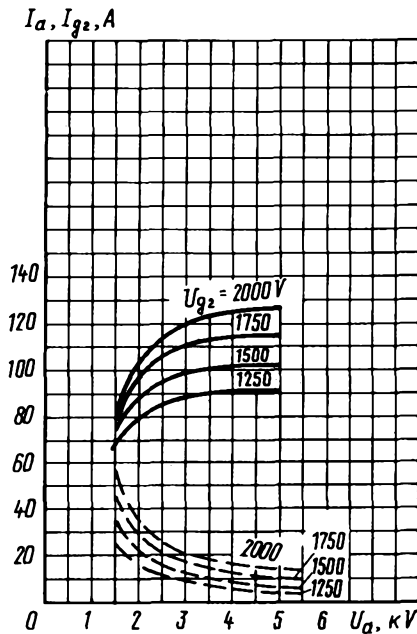
Усредненные характеристики: избыточное напряжение сетки первой в импульсе ( U_{g1} ) равно 125 В; — анодные; --- сеточно-анодные (по сетке первой)
