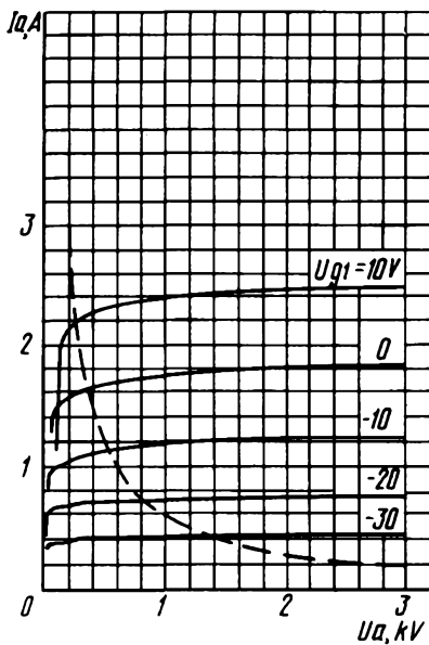
Усредненные анодные характеристики: U_i = 12,6 \text{ В}; U_{g2} = 300 \text{ В}; - - - - - наибольшая мощность, рассеиваемая анодом ( P_{a,max} )
