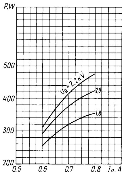
Характеристики зависимости полезной мощности от тока анода: U_g = 12,6 \text{ В}; \lambda = 30 \text{ см} Characteristic Curves Showing Output Power versus Anode Current: U_g = 12.6 \text{ V}; \lambda = 30 \text{ cm}
