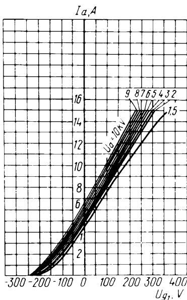
Усредненные анодно-сеточные характеристики: U_i = 6,3 \text{ В}; U_{g2} = 1,5 \text{ кВ} Averaged Anode-Grid Characteristic Curves: U_i = 6.3 \text{ V}; U_{g2} = 1.5 \text{ kV}
