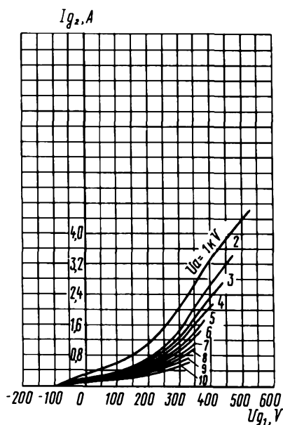
Усредненные сеточные характеристики (по сетке второй): U_i = 6.3 \text{ В}; U_{g2} = 1 \text{ кВ}
