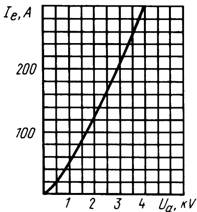
Усредненная эмиссионная характеристика: U_i = 6.3 \text{ V} Averaged Emission Characteristic Curves: U_i = 6.3 \text{ V}
