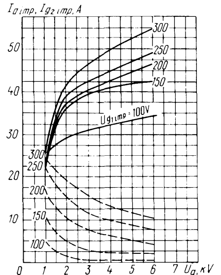
Усредненные импульсные характеристики: U_{g2} = 1 \text{ кВ}; — анодные; - - - сеточно-анодные (по сетке второй) Averaged Peak Characteristic Curves: U_{g2} = 1 \text{ kV}; — anode; - - - grid 2-anode
