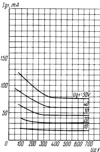
Усредненные сеточно-анодные характеристики (для одного тетрода): U_i = 6,3 \text{ В}; U_{g2} = 250 \text{ В} Averaged Grid-Anode Characteristic Curves (Each Tetraode): U_i = 6.3 \text{ V}; U_{g2} = 250 \text{ V}
