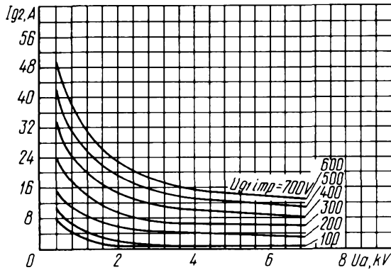
Усредненные импульсные сеточно-анодные характеристики (по сетке второй): U_1 = 9.5 \text{ В}; U_{q2} = 1 \text{ кВ} Averaged Peak Grid 2-Anode Characteristic Curves: U_1 = 9.5 \text{ V}; U_{q2} = 1 \text{ kV}
