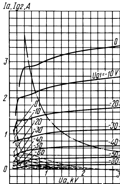
Усредненные характеристики: U_i = 12,6 \text{ В}; U_{g2} = 400 \text{ В}; U_{g3} = 0 \text{ В}; ————— анодные; - - - - - сеточно-анодные (по сетке второй); - · - · - · наибольшая мощность, рассеиваемая анодом ( P_{a \text{ max}} )
