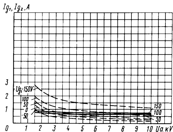
Усредненные характеристики: U_f = 8,3 В; U_{g2} = 1,5 кВ; — сеточно-анодные (по сетке первой); - - - сеточно-анодные (по сетке второй) Averaged Characteristic Curves: U_f = 8.3 V; U_{g2} = 1.5 kV; — grid 1-anode; - - - grid 2-anode
