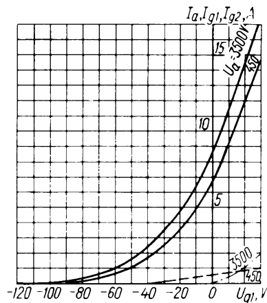
Усредненные характеристики: U_1 = 12,6 \text{ В}; U_{g2} = 400 \text{ В}; — анодно-сеточные; - - - сеточные по второй сетке; - · - · сеточные по первой сетке
