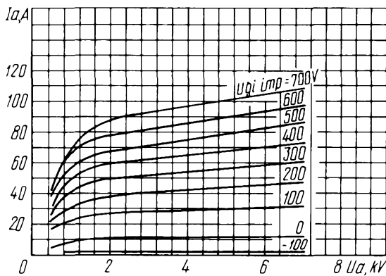
Усредненные импульсные анодные характеристики: U_1 = 9.5 \text{ В}; U_{q2} = 1 \text{ кВ} Averaged Peak Anode Characteristic Curves: U_1 = 9.5 \text{ В}; U_{q2} = 1 \text{ кВ}
