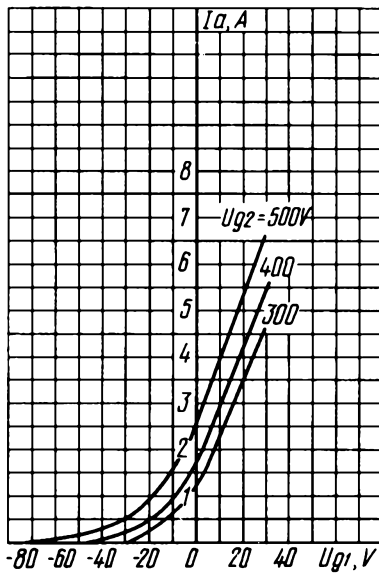
Усредненные анодно-сеточные характеристики:
