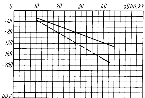
Усредненные характеристики запирающего: U_f = 26 В; I_a = 1 мА; — напряжение запирающего ( U_{g\text{ cutoff}} ); - - - напряжение смещения ( U_{gb} ) Averaged Cut-Off Characteristic Curves: U_f = 26 V; I_a = 1 mA; — cutoff voltage ( U_{g\text{ cutoff}} ); - - - bias voltage U_{gb}
