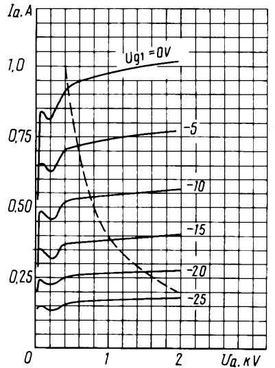
Усредненные анодные характеристики: U_i = 6,3 \text{ В}; U_{g2} = 325 \text{ В}; ——— ток анода ( I_a ); - - - - наибольшая мощность, рассеиваемая анодом ( P_{a \text{ max}} ) Averaged Anode Characteristic Curves: U_i = 6.3 \text{ V}; U_{g2} = 325 \text{ V}; ——— I_a ; - - - - P_{a \text{ max}}
