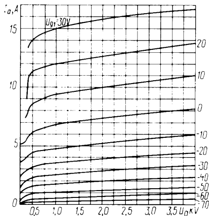
Усредненные анодные характеристики: U_1 = 12,6 \text{ В}; U_{g2} = 400 \text{ В}
