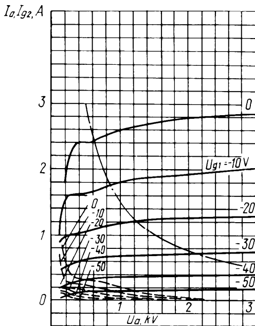
Усредненные характеристики: U_i = 12,6 \text{ В}; U_{g2} = 350 \text{ В}; U_{g3} = 0; ————— анодные; - - - - - сеточно-анодные (по сетке второй); - · - · - · наибольшая мощность, рассеиваемая анодом ( P_{a \text{ max}} )
