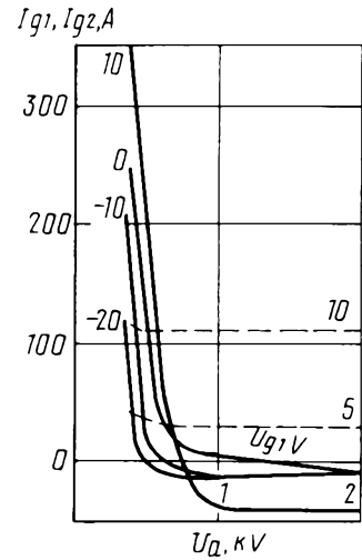
Усредненные характеристики: U_1 = 6 \text{ В}; U_{g2} = 400 \text{ В}; — — — сеточно-анодные (по сетке второй); - - - - сеточно-анодные (по сетке первой) Averaged Characteristic Curves: U_1 = 6 \text{ V}; U_{g2} = 400 \text{ V}; — — — grid 2-anode; - - - - grid 1-anode
