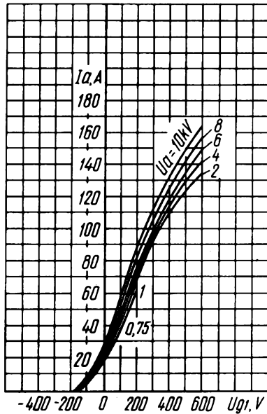
Усредненные анодно-сеточные характеристики: U_i = 22 \text{ В}; U_{g2} = 750 \text{ В} Averaged Anode-Grid Characteristic Curves: U_i = 22 \text{ V}; U_{g2} = 750 \text{ V}
