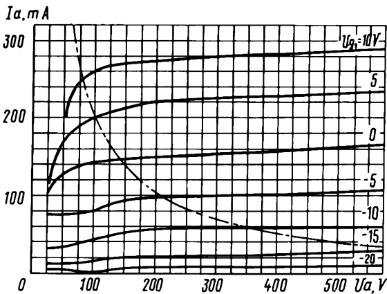
Усредненные анодные характеристики (каждого тетрода): U_1 = 12.6 \text{ В}; U_{g2} = 200 \text{ В}; — — — — — наибольшая мощность, рассеиваемая анодом ( P_{a \text{ макс}} )
