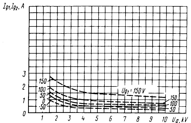
Усредненные характеристики: U_i = 8,3 \text{ В}; U_{g2} = 1,5 \text{ кВ}; — сеточно-анодные (по сетке первой); - - - сеточно-анодные (по сетке второй) Averaged Characteristic Curves: U_i = 8.3 \text{ V}; U_{g2} = 1.5 \text{ kV}; — grid 1-anode; - - - grid 2-anode
