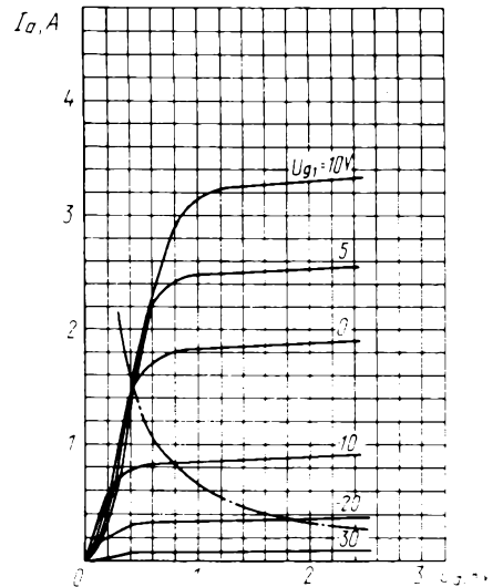
Усредненные анодные характеристики: U_1 = 12,6 \text{ В}; U_{g2} = 300 \text{ В}; — — — — — наибольшая мощность, рассеиваемая анодом ( P_{a \text{ max}} ) Averaged Anode Characteristic Curves: U_1 = 12.6 \text{ V}; U_{g2} = 300 \text{ V}; — — — — — P_{a \text{ max}}
