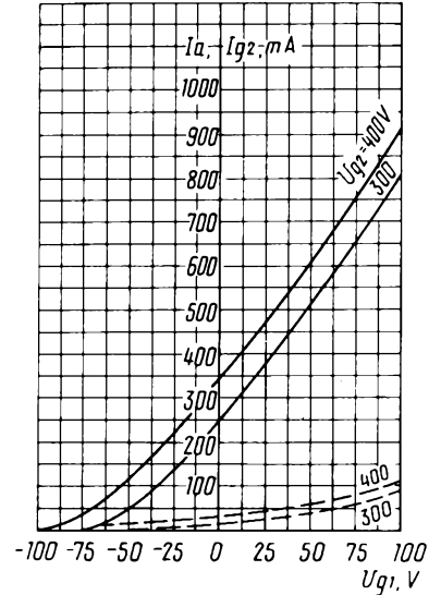
Усредненные характеристики: U_1 = 20 В; U_a = 1,5 кВ; U_{g3} = 50 В — — — — — анодно-сеточные; - - - - - сеточные (по сетке второй) Averaged Characteristic Curves: U_1 = 20 V; U_a = 1.5 kV; U_{g3} = 50 V — — — — — anode-grid; - - - - - grid 2
