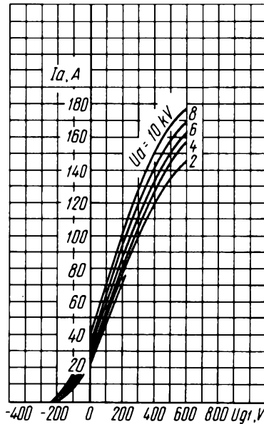
Усредненные анодно-сеточные характеристики: U_i = 22 \text{ В}; U_{g2} = 1000 \text{ В} Averaged Anode-Grid Characteristic Curves: U_i = 22 \text{ V}; U_{g2} = 1,000 \text{ V}
