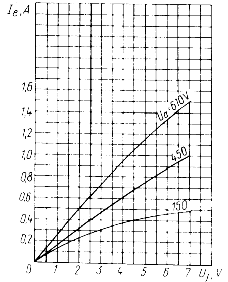
Типовая анодная характеристика: U_i = 5 \text{ V} ; \tau_{\text{imp}} = 1 \text{ мкс} ; частота посылок ( f_i ) равна 200 Гц Standard Anode Characteristic Curves: U_i = 5 \text{ V} ; \tau_{\text{imp}} = 1 \mu\text{s} ; pulse frequency 200 Hz
