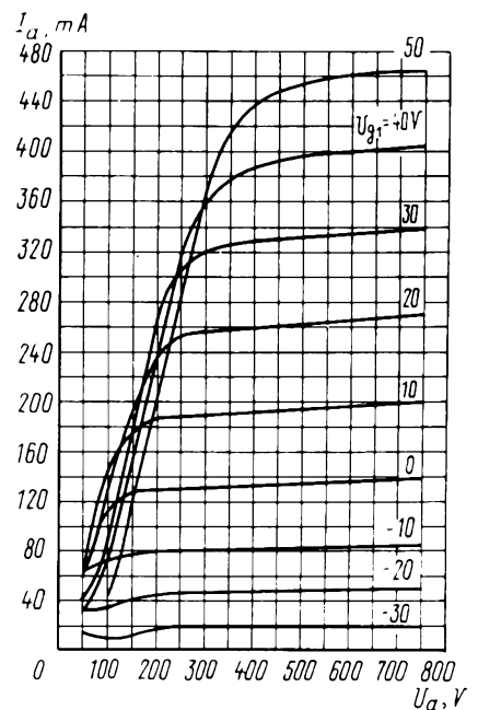
Усредненные анодные характеристики (для одного тетрода): U_i = 6,3 В; U_{g2} = 300 В Averaged Anode Characteristic Curves (Each Tetrode): U_i = 6.3 V; U_{g2} = 300 V
