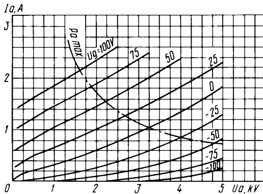
Усредненные анодные характеристики: U_f = 6,3 В; — — — — — наибольшая допустимая мощность, рассеиваемая анодом ( P_{a \max} ) Averaged Anode Characteristic Curves: U_f = 6.3 V; - - - - - P_{a \max}
