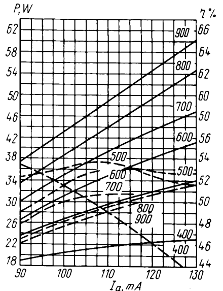
Усредненные характеристики в режиме автогенерации: U_i = 6,3 В; \lambda = 30 см; — колебательная мощность (P); --- коэффициент полезного действия ( \eta ) Averaged Characteristic Curves for Oscillation Mode: U_i = 6.3 V; \lambda = 30 cm; — oscillator output power (P); --- efficiency ( \eta )
