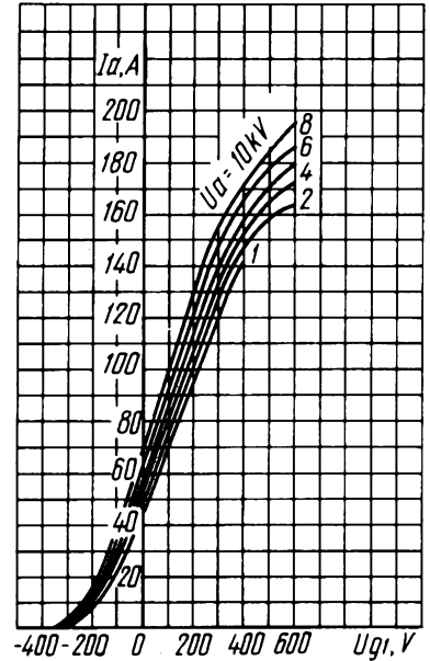
Усредненные анодно-сеточные характеристики: U_i = 22 \text{ В}; U_{g2} = 1500 \text{ В} Averaged Anode-Grid Characteristic Curves: U_i = 22 \text{ V}; U_{g2} = 1,500 \text{ V}
