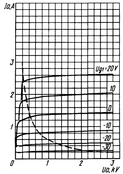
Усредненные анодные характеристики: U_i = 12,6 \text{ В}; U_{g2} = 250 \text{ В}; - - - - - наибольшая мощность, рассеиваемая анодом ( P_{a,max} )
