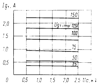
Усредненные импульсные сеточно-анодные характеристики (по сетке первой): U_i = 12,6 В; U_{g2} = 500 В Averaged Peak Grid 1-Anode Characteristic Curves: U_i = 12.6 V; U_{g2} = 500 V
