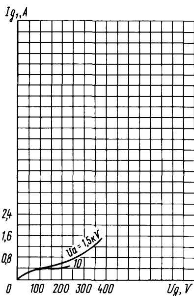
Усредненные сеточные характеристики (по сетке первой): U_i = 6.3 \text{ В}; U_{g2} = 1.5 \text{ кВ}
