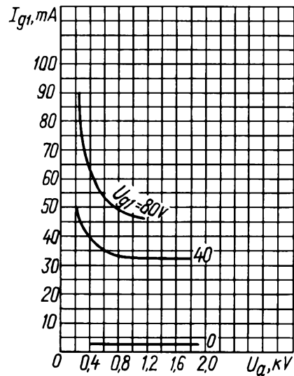
Усредненные сеточно-анодные характеристики: U_1 = 12.6 \text{ В}; U_{g2} = 0.5 \text{ кВ} Averaged Grid-Anode Characteristic Curves: U_1 = 12.6 \text{ V}; U_{g2} = 0.5 \text{ kV}
