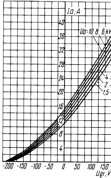
Усредненные анодно-сеточные характеристики: U_i = 8,3 \text{ В}; U_{g2} = 1 \text{ кВ} Averaged Anode-Grid Characteristic Curves: U_i = 8.3 \text{ V}; U_{g2} = 1 \text{ kV}
