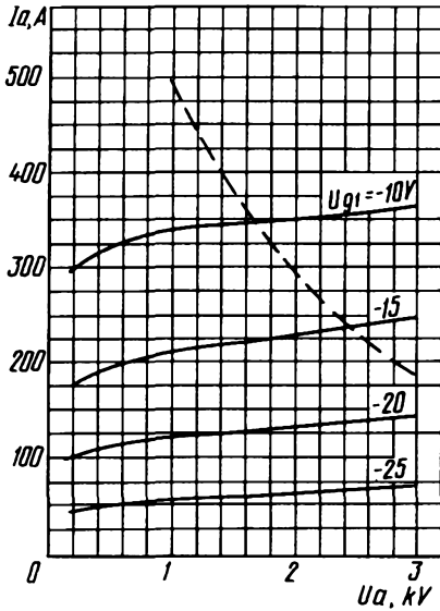
Усредненные анодные характеристики: U_i = 12,6 \text{ В}; U_{g2} = 150 \text{ В}; - - - - - наибольшая мощность, рассеиваемая анодом ( P_{a,max} )
