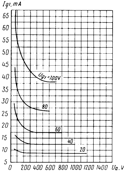
Усредненные сеточно-анодные характеристики: U_1 = 20 В; U_{g2} = 0,4 кВ; U_{g3} = 50 В Averaged Grid-Anode Characteristic Curves: U_1 = 20 V; U_{g2} = 0.4 kV; U_{g3} = 50 V
