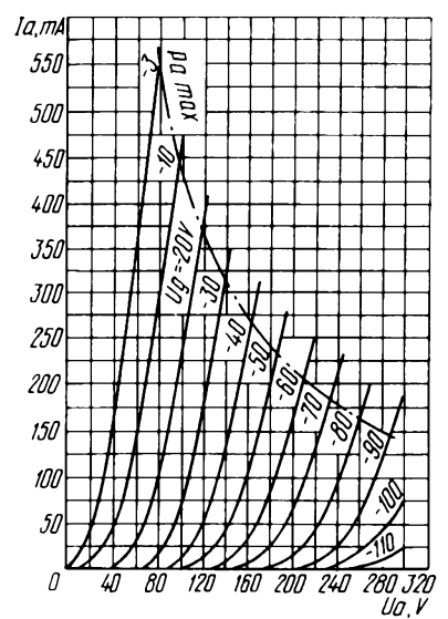
Усредненные анодные характеристики (при работе с одним катодом): U_f = 6,3 В; — — — наибольшая допустимая мощность, рассеиваемая анодом ( P_{a \max} ) Averaged Anode Characteristic Curves (single-cathode operation): U_f = 6.3 V; - - - - P_{a \max}
