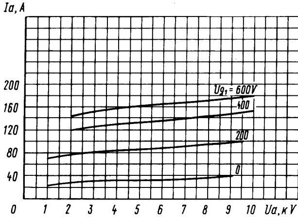
Усредненные анодные характеристики: U_i = 22 \text{ В}; U_{g2} = 1500 \text{ В} Averaged Characteristic Curves: U_i = 22 \text{ V}; U_{g2} = 1,500 \text{ V}
