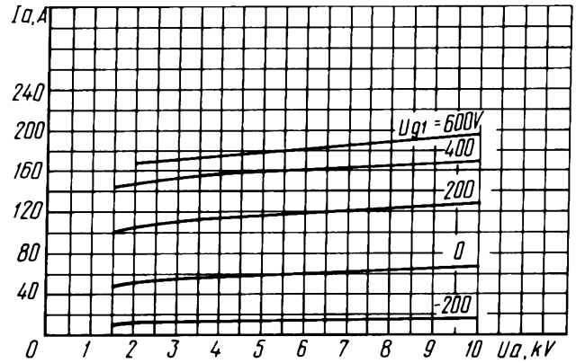
Усредненные анодные характеристики: U_i = 22 \text{ В}; U_{g2} = 1000 \text{ В} Averaged Anode Characteristic Curves: U_i = 22 \text{ V}; U_{g2} = 1,000 \text{ V}
