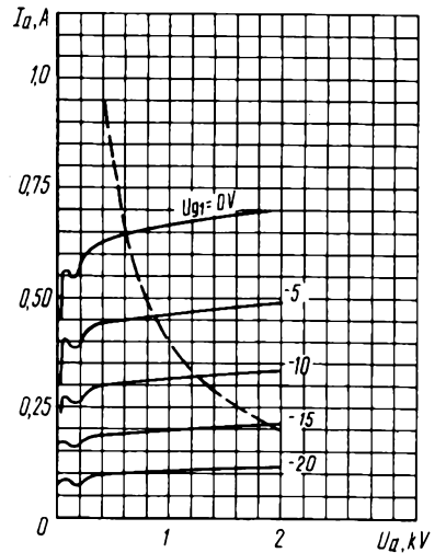
Усредненные анодные характеристики: U_i = 6,3 \text{ В}; U_{g2} = 250 \text{ В}; ток анода ( I_a ); --- наибольшая мощность, рассеиваемая анодом ( P_{a \text{ max}} ) Averaged Anode Characteristic Curves: U_i = 6.3 \text{ V}; U_{g2} = 250 \text{ V}; ——— I_a ; - - - - P_{a \text{ max}}
