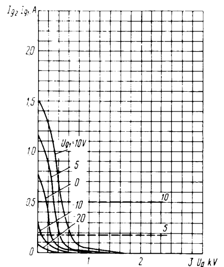
Усредненные характеристики: U_1 = 12,6 \text{ В}; U_a = 100 \text{ В}; — — — — — анодно-сеточные; - - - - - сеточные (по сетке второй); - - - - - сеточные (по сетке первой) Averaged Characteristic Curves: U_1 = 12.6 \text{ V}; U_a = 1,000 \text{ V}; — — — — — anode-grid; - - - - - grid 2; - - - - - grid 1
