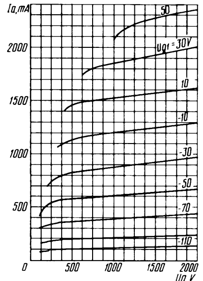
Усредненные анодные характеристики: U_i = 8,3 В; U_{g2} = 0,6 кВ; U_{g3} = 0 В Averaged Anode Characteristic Curves: U_i = 8.3 V; U_{g2} = 0.6 kV; U_{g3} = 0 V
