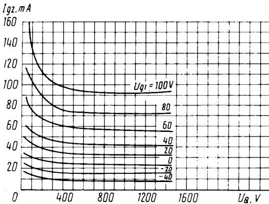
Усредненные анодные характеристики: — — — — — наибольшая мощность, рассеиваемая анодом ( P_{a,max} ); U_1 = 20 В; U_{g2} = 0,4 кВ; U_{g3} = 50 В Averaged Anode Characteristics: U_1 = 20 V; U_{g2} = 0.4 kV; U_{g3} = 50 V; - - - - - P_{a,max}
