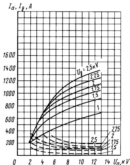
Усредненные характеристики: U_f = 26 В; — ток анода ( I_a ); - - - ток сетки ( I_g ) Averaged Characteristic Curves: U_f = 26 В; — I_a ; - - - I_g
