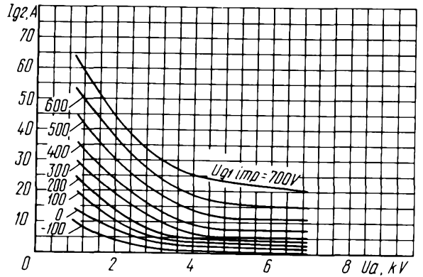
Усредненные импульсные сеточно-анодные характеристики (по сетке второй): U_1 = 9.5 \text{ В}; U_{q2} = 2.5 \text{ кВ} Averaged Peak Grid 2-Anode Characteristic Curves: U_1 = 9.5 \text{ В}; U_{q2} = 2.5 \text{ кВ}
