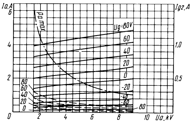
Усредненные характеристики: U_f = 5 \text{ В} ; U_{g2} = 800 \text{ В} ; ——— анодные; - - - - сеточно-анодные; - · - · наибольшая мощность, рассеиваемая анодом ( P_{a \text{ max}} ) Averaged Characteristic Curves: U_f = 5 \text{ V} ; U_{g2} = 800 \text{ V} ; ——— anode; - - - - grid-anode; - · - · P_{a \text{ max}}
