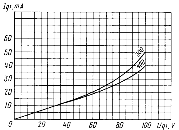
Усредненные сеточные характеристики: U_1 = 20 В; U_a = 1,5 кВ; U_{g3} = 50 В
