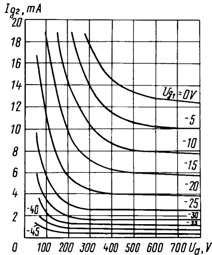
Усредненные сеточно-анодные характеристики (по второй сетке): U_i = 12,6 V; U_{g2} = 250 V; U_{g3} = 0 V Averaged Grid 2-Anode Characteristic Curves: U_i = 12.6 V; U_{g2} = 250 V; U_{g3} = 0
