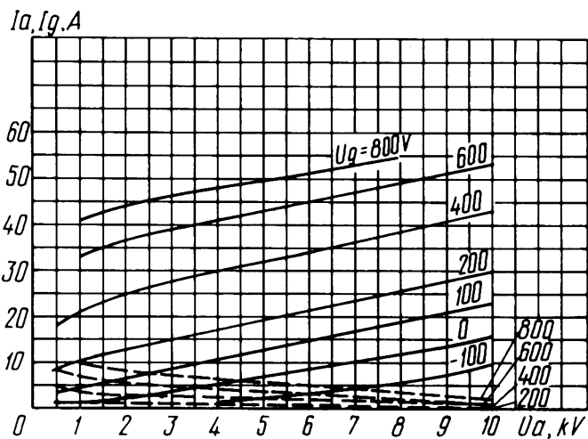
Усредненные характеристики: U_f = 8,3 \text{ В} ; — анодные; - - - сеточно-анодные Averaged Characteristic Curves: U_f = 8.3 \text{ V} — anode; - - - grid-anode
