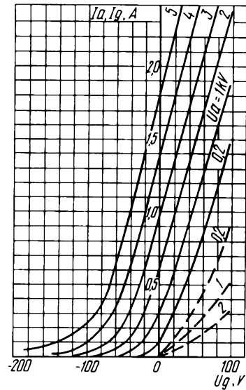
Усредненные характеристики: U_f = 6,3 В; — — — — — анодно-сеточные; - - - - - сеточные Averaged Characteristic Curves: U_f = 6.3 V; - - - - - anode-grid; - - - - - grid
