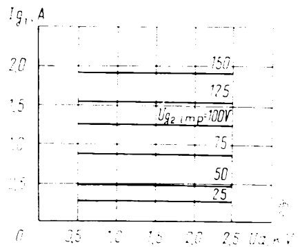
Усредненные импульсные сеточно-анодные характеристики (по сетке первой): U_i = 12,6 В; U_{g2} = 600 В Averaged Peak Grid 1-Anode Characteristic Curves: U_i = 12.6 V; U_{g2} = 600 V
