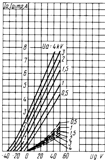
Усредненные импульсные характеристики: U_i = 6,3 В; \tau = 1 мкс; частота посылок ( f_i ) равна 1000 Гц; ————— анодные; - - - - - сеточные Averaged Peak Characteristic Curves: U_i = 6.3 V; \tau = 1 \mu s; pulse frequency 1,000 Hz; ————— anode; - - - - - grid
