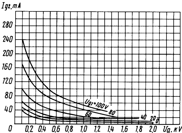
Усредненные сеточно-анодные характеристики (по сетке второй): U_i = 10 \text{ В}; U_{g2} = 0.3 \text{ кВ}; напряжение лучеобразующих пластин ( U_{пн} ) равно 0 В Averaged Grid 2-Anode Characteristic Curves: U_i = 10 \text{ V}; U_{g2} = 0.3 \text{ kV}; beam-forming plates voltage U_{пн} is 0
