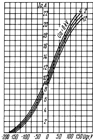
Усредненные анодно-сеточные характеристики: U_1 = 8.3 \text{ В}; U_{q2} = 1.2 \text{ кВ} Averaged Anode-Grid Characteristic Curves: U_1 = 8.3 \text{ V}; U_{q2} = 1.2 \text{ kV}
