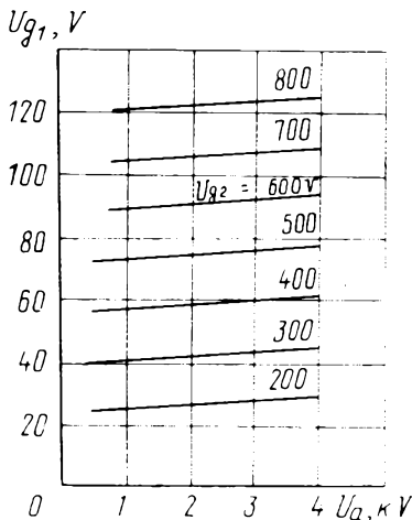
Характеристики зависимости напряжения записания от напряжения анода и второй сетки: U_i = 12,6 В; I_a = 0,2 мА Characteristic Curves Showing Cutoff Voltage versus Anode and Grid 2 Voltages: U_i = 12.6 V; I_a = 0.2 mA
