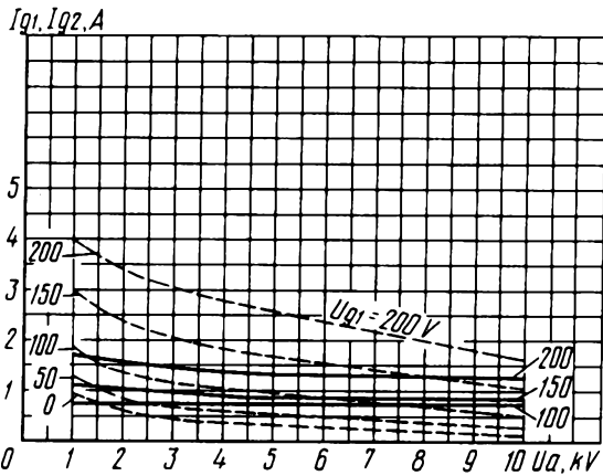
Усредненные характеристики: U_i = 8,3 \text{ В}; U_{g2} = 1 \text{ кВ}; — сеточно-анодные (по сетке первой); - - - сеточно-анодные (по сетке второй) Averaged Characteristic Curves: U_i = 8.3 \text{ V}; U_{g2} = 1 \text{ kV}; — grid 1-anode; - - - grid 2-anode
