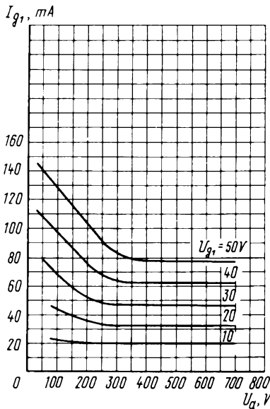
Усредненные сеточно-анодные характеристики (для одного тетрода): U_i = 6,3 \text{ В}; U_{g2} = 200 \text{ В} Averaged Grid-Anode Characteristic Curves (Each Tetraode): U_i = 6.3 \text{ V}; U_{g2} = 200 \text{ V}
