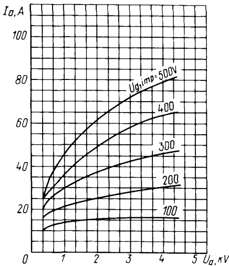
Усредненные импульсные анодные характеристики: U_1 = 9.5 \text{ В}; U_{q2} = 400 \text{ В} Averaged Peak Anode Characteristic Curves: U_1 = 9.5 \text{ В}; U_{q2} = 400 \text{ В}
