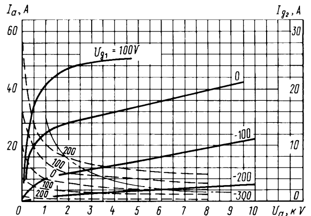
Усредненные характеристики: U_f = 14 \text{ В}; U_{g2} = 1,75 \text{ кВ}; ——— анодные; - - - - - сеточно-анодные; - · - · - · наибольшая допустимая мощность, рассеиваемая анодом ( P_{a \text{ max}} )
