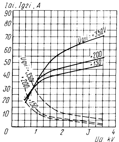
Усредненные импульсные характеристики:
