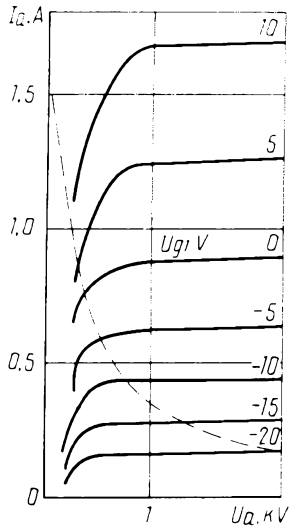
Усредненные анодные характеристики: U_1 = 6 \text{ В}; U_{g2} = 400 \text{ В}; — — — наибольшая мощность, рассеиваемая анодом ( P_{a \text{ max}} ) Averaged Anode Characteristic Curves: U_1 = 6 \text{ V}; U_{g2} = 400 \text{ V}; — — — P_{a \text{ max}}
