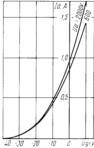
Усредненные анодно-сеточные характеристики: U_1 = 6 \text{ В}; U_{g2} = 400 \text{ В} Averaged Anode-Grid Characteristic Curves: U_1 = 6 \text{ V}; U_{g2} = 400 \text{ V}
