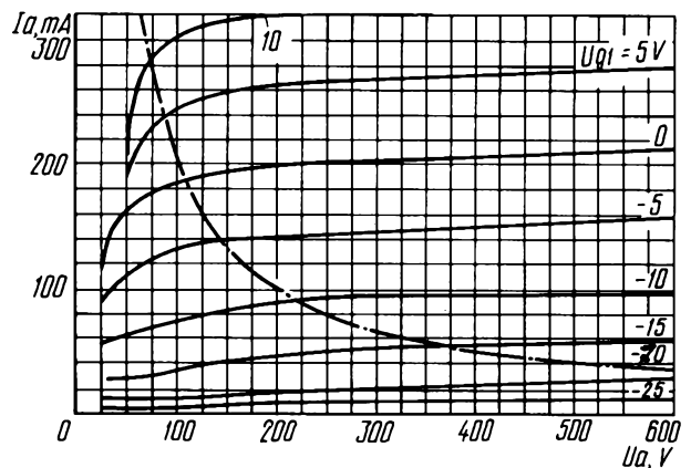
Усредненные анодные характеристики (каждого тетрода): U_1 = 12.6 \text{ В}; U_{g2} = 250 \text{ В}; — — — — — наибольшая мощность, рассеиваемая анодом ( P_{a \text{ макс}} )
