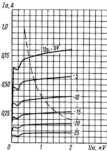
Усредненные анодные характеристики: U_i = 6,3 \text{ В}; U_{g2} = 275 \text{ В}; ——— ток анода ( I_a ); - - - - наибольшая мощность, рассеиваемая анодом ( P_{a \text{ max}} ) Averaged Anode Characteristic Curves: U_i = 6.3 \text{ V}; U_{g2} = 275 \text{ V}; ——— I_a ; - - - - P_{a \text{ max}}
