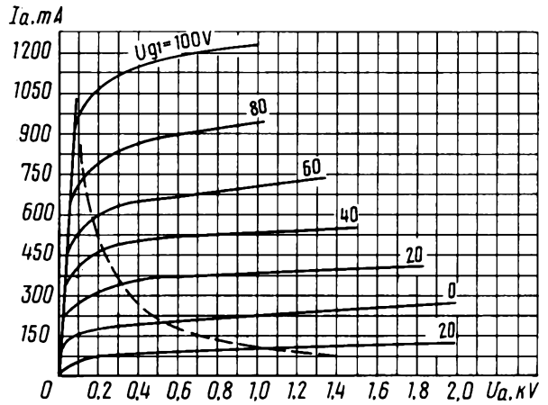
Усредненные анодные характеристики: U_i = 10 \text{ В}; U_{g2} = 0.4 \text{ кВ}; — — — наибольшая мощность, рассеиваемая анодом ( P_{a \text{ max}} ); напряжение лучеобразующих пластин ( U_{пн} ) равно 0 В Averaged Anode Characteristic Curves: U_i = 10 \text{ V}; U_{g2} = 0.4 \text{ kV}; — — — P_{a \text{ max}} beam-forming plates voltage U_{пн} is 0
