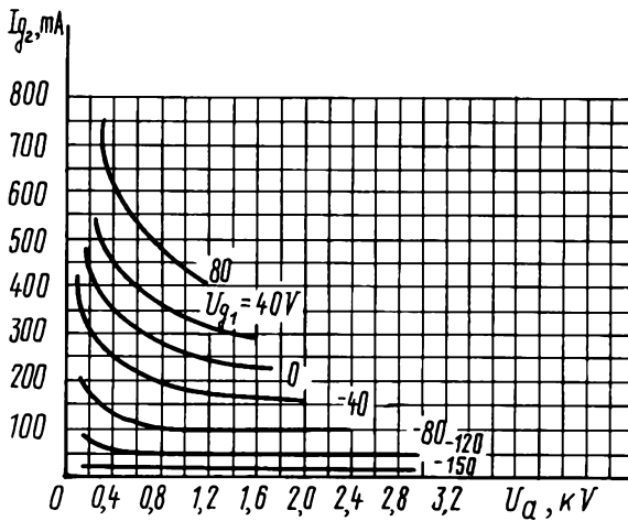
Усредненные сеточно-анодные характеристики по второй сетке: U_1 = 12.6 \text{ В}; U_{g2} = 0.6 \text{ кВ} Averaged Characteristic Curves: U_1 = 12.6 \text{ V}; U_{g2} = 0.6 \text{ kV}
