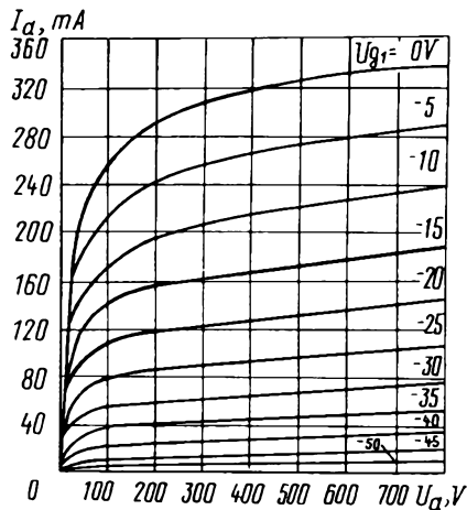
Усредненные анодные характеристики (по сетке второй): U_i = 12,6 V; U_{g2} = 250 V; U_{g3} = 0 V Averaged Anode-Grid 2 Characteristic Curves: U_i = 12.6 V; U_{g2} = 250 V; U_{g3} = 0
