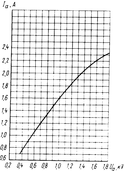
Типовая анодная характеристика: U_i = 5 \text{ V} ; \tau_{\text{imp}} = 1 \text{ мкс} ; частота посылок ( f_i ) равна 200 Гц Standard Anode Characteristic Curves: U_i = 5 \text{ V} ; \tau_{\text{imp}} = 1 \mu\text{s} ; pulse frequency 200 Hz
