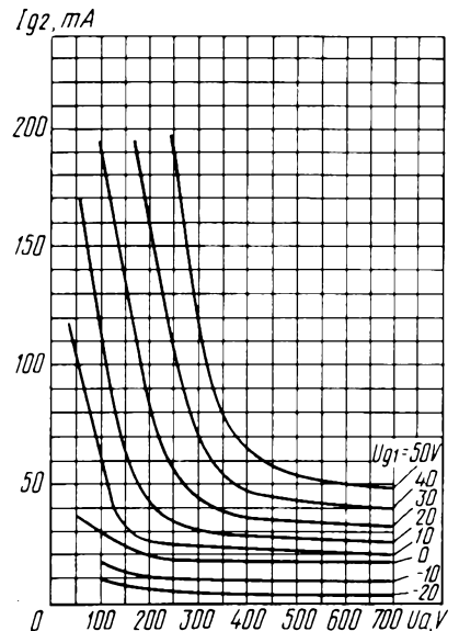
Усредненные сеточно-анодные характеристики (для одного тетрода): U_i = 6,3 \text{ В}; U_{g2} = 250 \text{ В} Averaged Grid-Anode Characteristic Curves (Each Tetraode): U_i = 6.3 \text{ V}; U_{g2} = 250 \text{ V}
