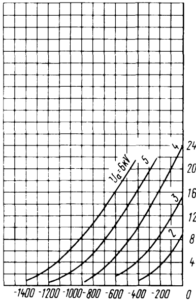
Усредненные анодно-сеточные характеристики: U_f = 10,5 \text{ В} Averaged Anode-Grid Characteristic Curves: U_f = 10.5 \text{ V}
