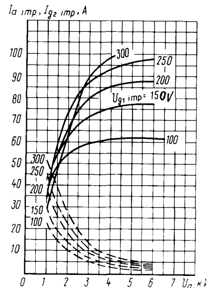
Усредненные импульсные характеристики: U_{g2} = 2,5 \text{ кВ}; — анодные; - - - анодно-сеточные (по сетке второй) Averaged Peak Characteristic Curves: U_{g2} = 2,5 \text{ kV}; — anode; - - - anode-grid 2
