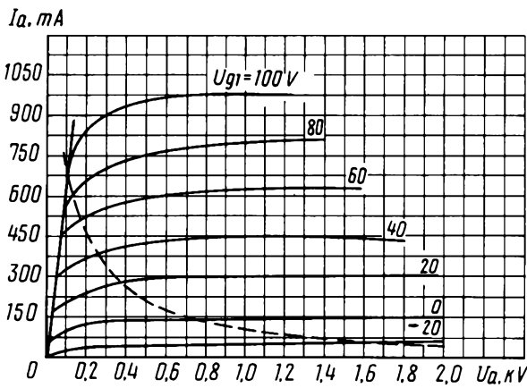
Усредненные анодные характеристики: U_i = 10 \text{ В}; U_{g2} = 0.3 \text{ кВ}; — — — наибольшая мощность, рассеиваемая анодом ( P_{a \text{ max}} ); напряжение лучеобразующих пластин ( U_{пн} ) равно 0 В Averaged Anode Characteristic Curves: U_i = 10 \text{ V}; U_{g2} = 0.3 \text{ kV}; — — — P_{a \text{ max}} beam-forming plates voltage U_{пн} is 0
