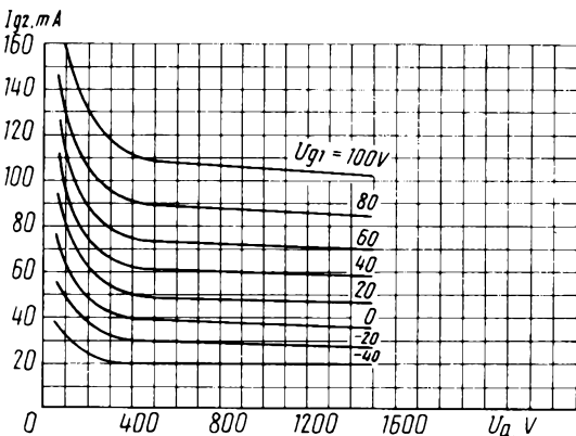
Усредненные сеточно-анодные характеристики (по сетке второй): U_1 = 20 В; U_{g2} = 0,4 кВ; U_{g3} = 50 В
