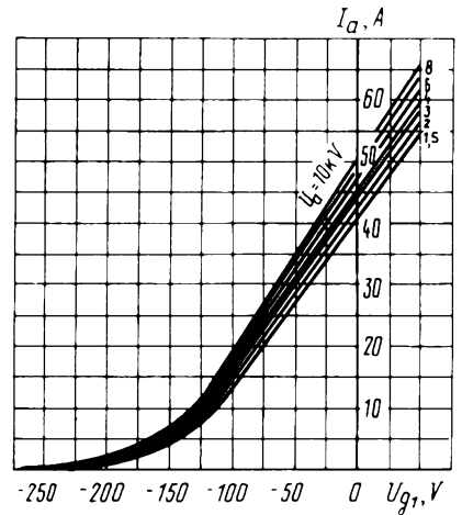
Усредненные анодно-сеточные характеристики: U_{g2} = 1500 V; U_i = 18 V Averaged Anode-Grid Characteristic Curves: U_i = 18 V; U_{g2} = 1,500 V
