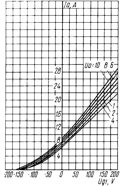
Усредненные анодно-сеточные характеристики: U_i = 8,3 \text{ В}; U_{g2} = 1,5 \text{ кВ} Averaged Anode Characteristic Curves: U_i = 8.3 \text{ V}; U_{g2} = 1.5 \text{ kV}
