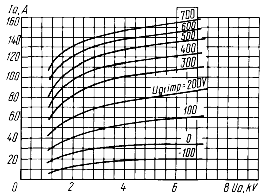
Усредненные импульсные анодные характеристики: U_1 = 9.5 \text{ В}; U_{q2} = 2.5 \text{ кВ} Averaged Peak Anode Characteristic Curves: U_1 = 9.5 \text{ В}; U_{q2} = 2.5 \text{ кВ}
