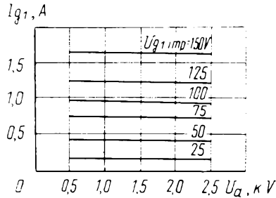
Усредненные импульсные сеточно-анодные характеристики (по сетке первой): U_1 = 12,6 В; U_{g2} = 700 В
