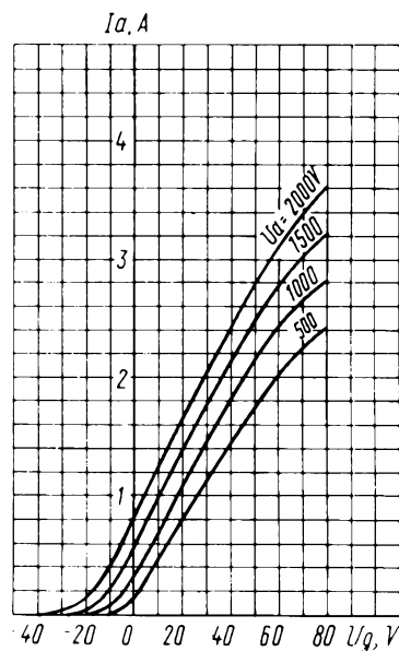
Усредненные импульсные анодно-сеточные характеристики: U_f = 6,3 В; \tau = 1 мкс; частота посылок ( f_p ) равна 2000 имп/с Averaged Anode-Grid Characteristic Curves in Pulsed Operation: U_f = 6.3 V; \tau = 1 \mu s; frequency 2,000 imp/s
