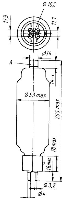
1 – катод; 2, 3 – не подключены; 4 – катод; A – анод – верхний вывод – колпачок; I – ключ
