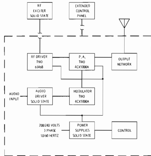
820E/F Diagram
