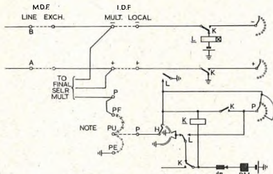
FIG. 8.—I.D.F. CONNEXIONS.
