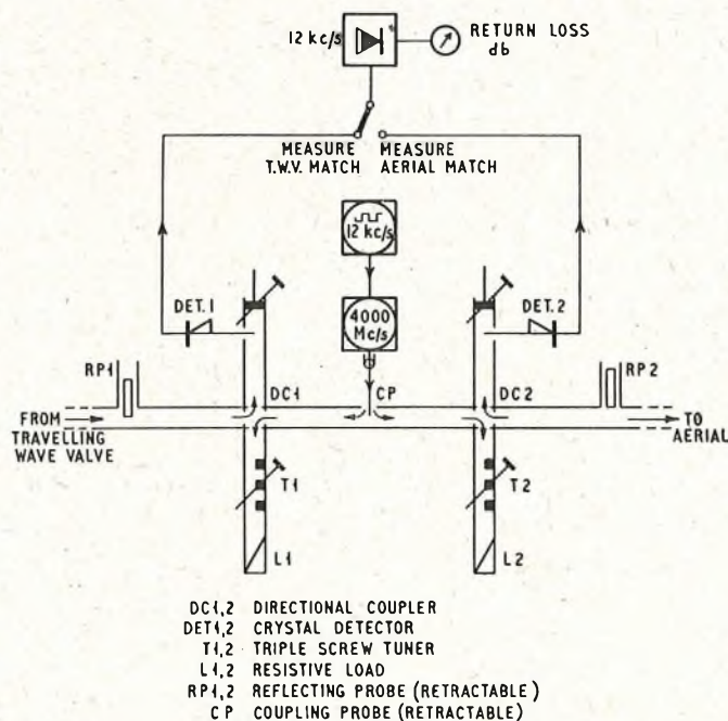
FIG. 18.—REFLECTOMETER.
