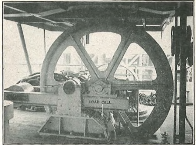
FIG. 3.—DYNAMOMETER SHEAVE.
