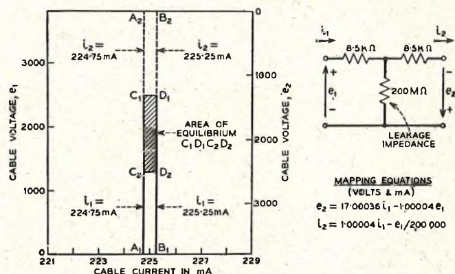
FIG. 9.—EQUILIBRIUM DIAGRAM.
