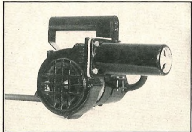
FIG. 8.—CABLE DRIER.
