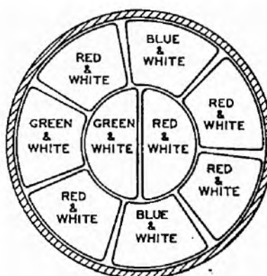
FIG. 1.—909-PAIR AMERICAN TYPE UNIT CABLE (4 LB.).
