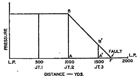
FIG. 1.—TYPE "A" FAULT.
