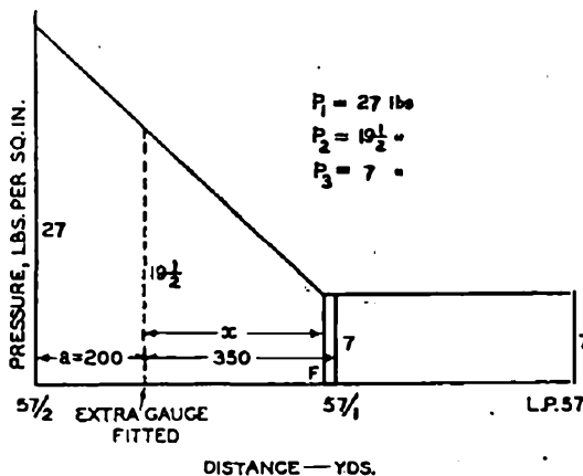
FIG. 2.—TYPE "B" FAULT.
