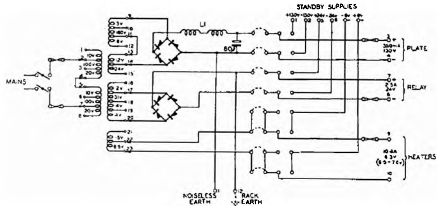
FIG. 5.—Mains Unit.
