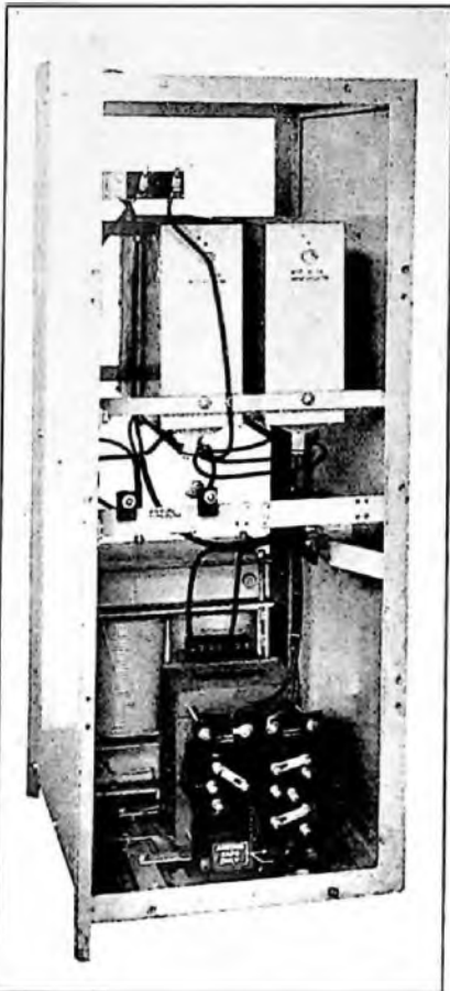
FIG. 3.—RECTIFIER No. 47E.
